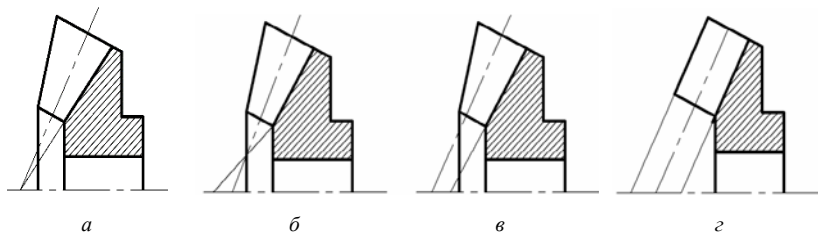
Рис. 1.7. Схема зубьев конических колес в зависимости от изменения размеров сечений по длине: a – форма I; б, в – форма II; г – форма III
