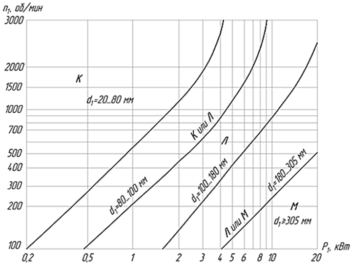
Рис. 7.5. Диаграмма для выбора сечения поликлинового ремня
