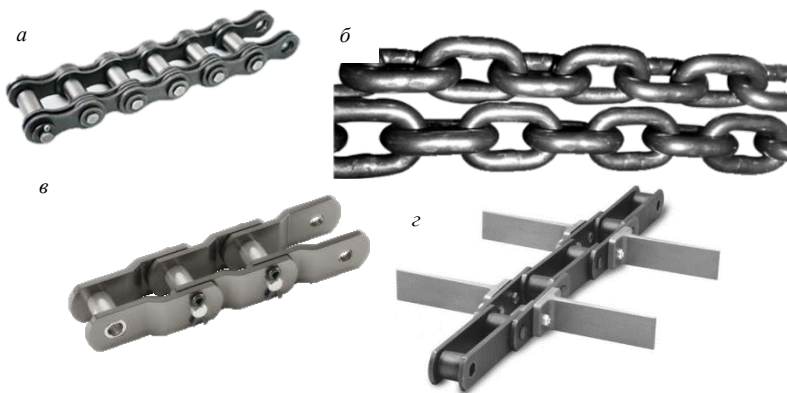
Рис. 8.1. Цепи грузовые и тяговые:
