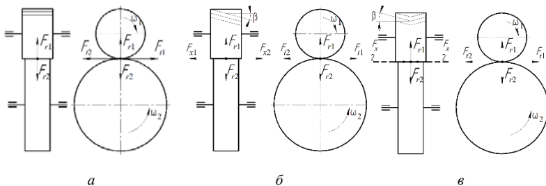
Рис. 3.1. Схема сил, действующих в цилиндрической передаче:
