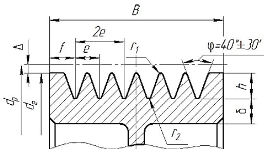
Рис. 7.7. Основные параметры шкива поликлиноременной передачи
