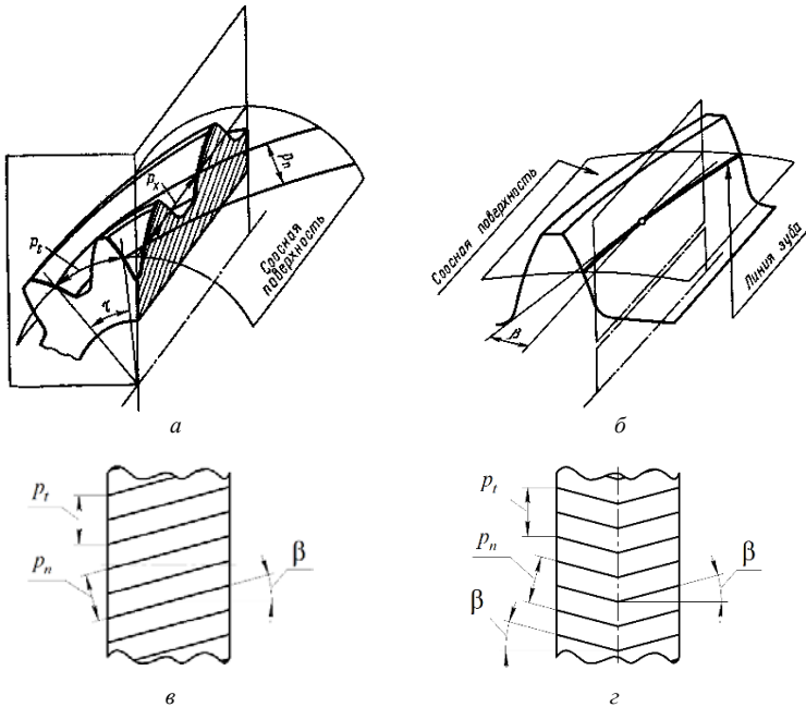
Рис. 1.4. Геометрические параметры зубчатых эвольвентных цилиндрических передач: а, б, в – для косозубых передач; г – для шевронных передач
