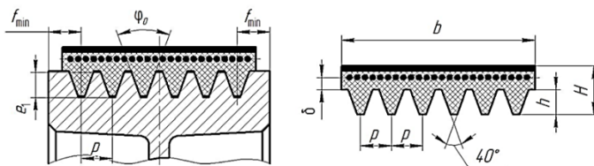
Рис. 7.6. Основные размеры поликлинового ремня
