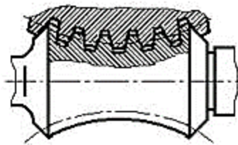
Рис. 5.8. Зацепление в глобоидной червячной передаче
