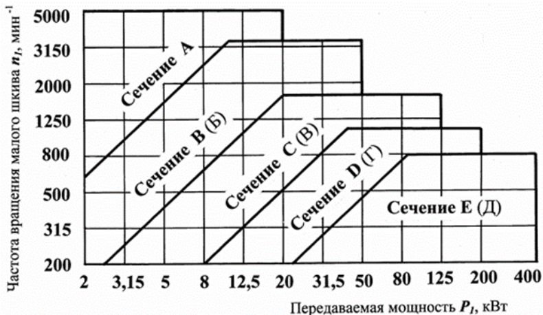
Рис. 7.2. Диаграмма для выбора сечения клинового ремня
