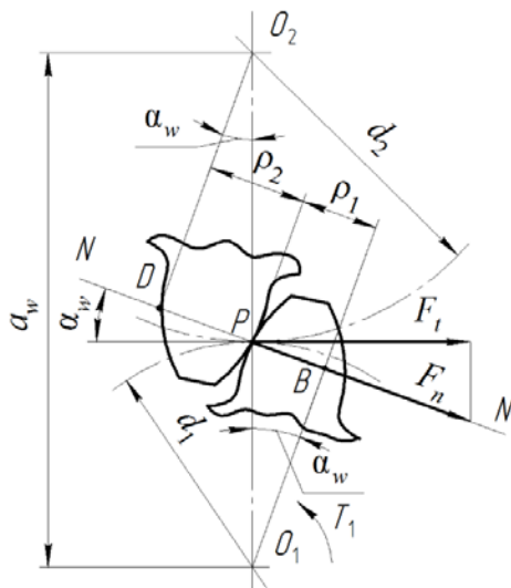
Рис. 2.2. Схема соприкосновения зубьев в полюсе зацепления
