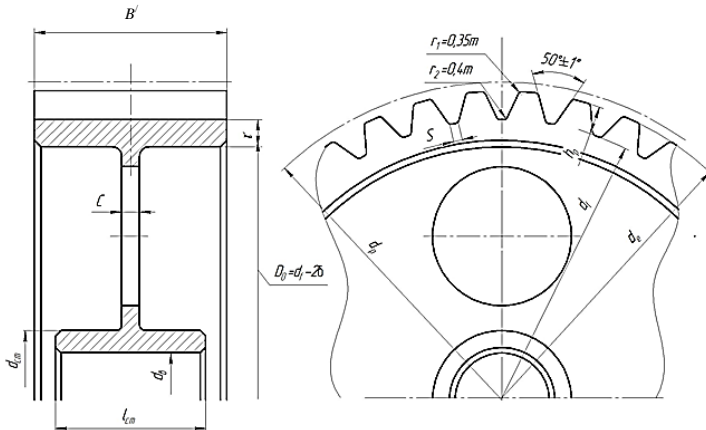
Рис. 7.9. Основные параметры шкивов зубчатого ремня
