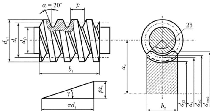
Рис. 5.4. Параметры червячной передачи
