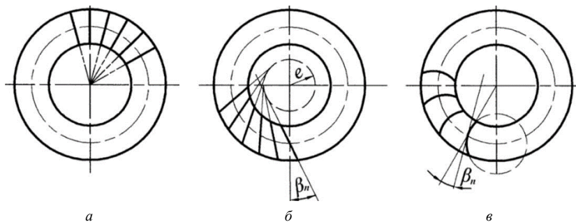
Рис. 1.6. Форма зубьев конического колеса: a – прямозубая; б – тангенциальная; в – с круговыми зубьями
