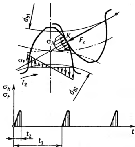
Рис. 2.1. Схема действия силы F_n на зуб цилиндрической передачи
