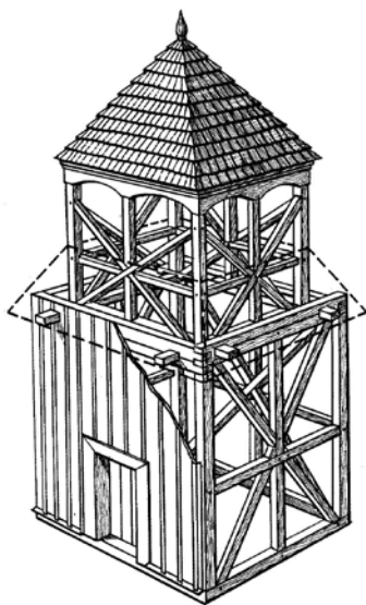
Рис. 15. Конструкция каркасной колокольни в д. Трокели Вороновского р-на, XVIII в.
