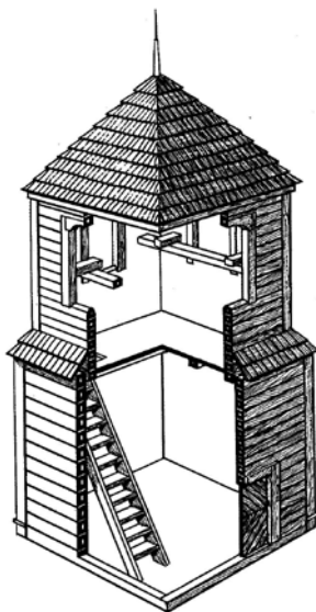
Рис. 16. Конструкция срубной колокольни в д. Дуды Ивьевского р-на, XVIII в.
