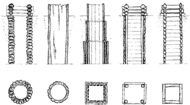
Рис. 22. Конструктивные типы колодезных проемов (по А. И. Локотко)
