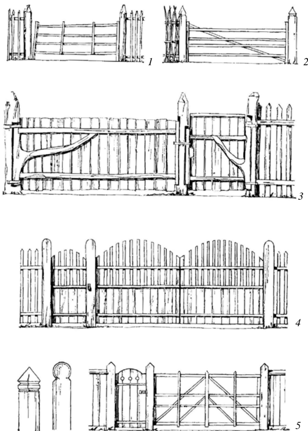
Рис. 19. Ворота XIX–XX вв. (по В. В. Трацевскому): 1 – г. п. Порозово Свислочского р-на; 2 – д. Крево Сморгонского р-на; 3 – д. Скрыгалово Мозырского р-на; 4 – Мозырский р-н; 5 – д. Юровичи Калинковичского р-на
