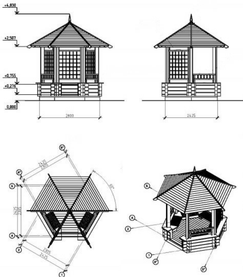
Рис. 44. Фрагмент чертежа деревянной беседки
