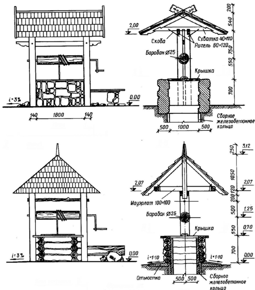
Рис. 42. Примеры колодцев с навесами
