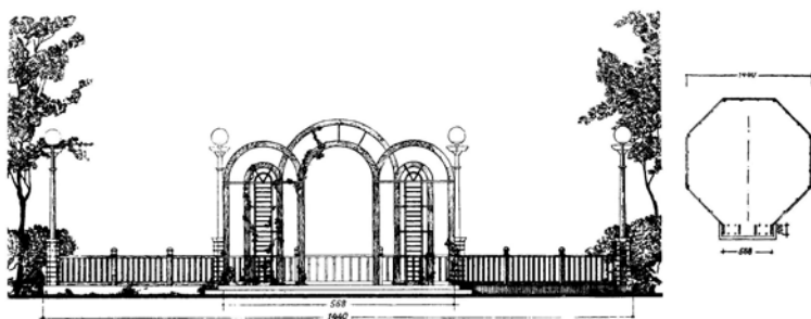
Рис. 27. Пример проектного предложения танцевальной площадки (фасад и план)
