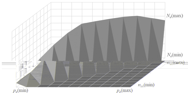
Рис. 1. Область режимов работы тракторного дизеля
