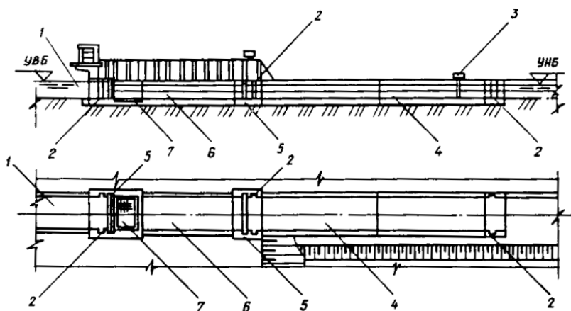
Рис. 1.17. Рыбопропускной шлюз:
