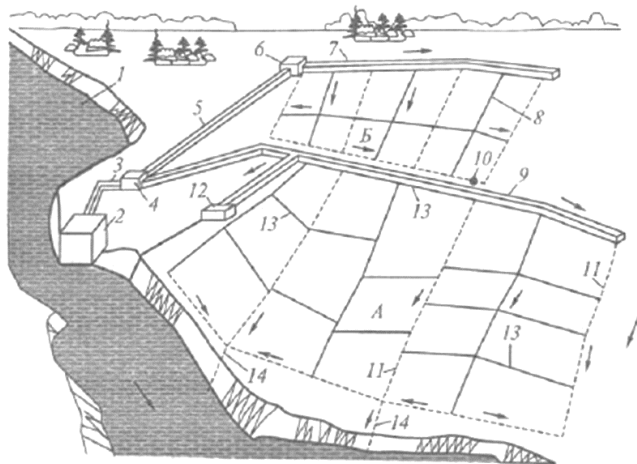
Рис. 1.8. Схема оросительной системы: А – зона самотечного орошения; Б – зона машинного орошения; 1 – река; 2 – головное сооружение; 3 – холостая часть магистрального канала; 4 – насосная станина; 5 – напорный трубопровод; 6 – открытый бассейн; 7 – ветвь магистрального канала; 8 – межхозяйственное распределение; 9 – рабочая часть магистрального канала; 10 – дюкер; 11 – водоотводящие каналы; 12 – ГЭС; 13 – внутрихозяйственные распределители; 14 – сбросной канал
