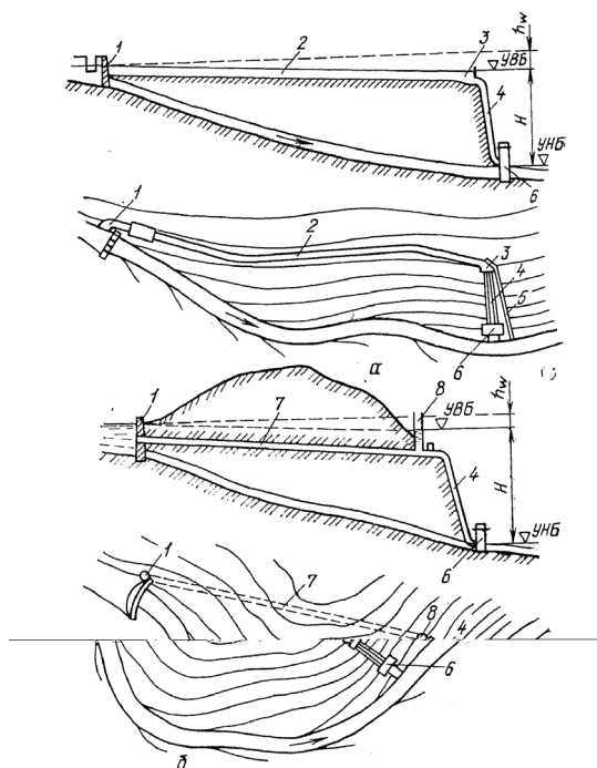
Рис. 1.26. Схемы деривационных ГЭС: а – с безнапорной деривацией; б – с напорной деривацией; 1 – головной водозаборный узел; 2 – деривационный канал; 3 – напорный бассейн; 4 – турбинный трубопровод; 5 – холостой водосброс; 6 – здание станции; 7 – напорный туннель; 8 – уравнильный резервуар
