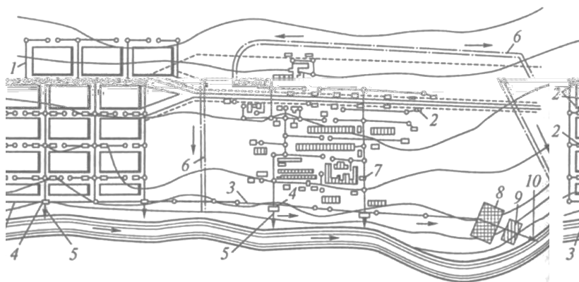
Рис. 1.4 Общесплавная система водоотведения: 1 – уличная сеть; 2 – дождеприемник; 3 – главный коллектор; 4 – ливнепуск; 5 – ливнеотвод; 6 – нагорная канава; 7 – заводская сеть; 8 – сооружения по очистке сточных вод; 9 – сооружения доочистки сточных вод; 10 – выпуск
