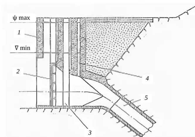
Рис. 1.41. Схема глубинного берегового водоприемника с засыпанной пазухой напорной стенки: 1 – забральная балка; 2 – сороудерживающая решетка; 3 – паз для затвора, 4 – воздухоподводящая труба; 5 – туннель
