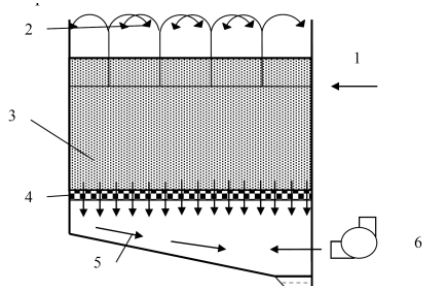
Рис. 2.1. Схема устройства биофильтра: 1 – подача сточных вод; 2 – водораспределительное устройство; 3 – слой фильтрующего материала; 4 – дренажное устройство; 5 – очищенная сточная вода; 6 – воздуханаспределительное устройство
