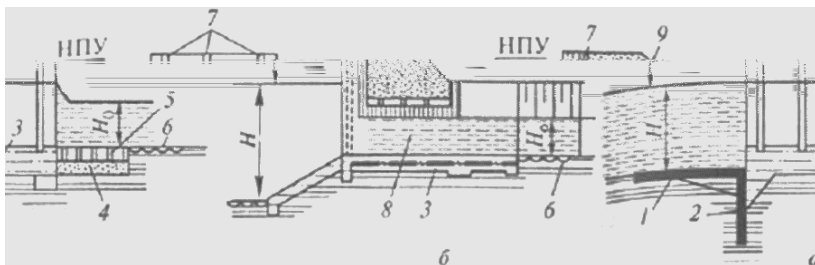
Рис. 1.9 Сооружения по оросительной сети: а – головной шлюз-регулятор открытого типа; б – трубчатый шлюз-регулятор закрытого типа; 1 – крепление понура; 2 – шпунт; 3 – водобойная часть; 4 – обратный фильтр; 5 – сквозной флютбет; 6 – крепление выходной части; 7 – пазы шандоров и затвора; 8 – труба; 9 – обратная засыпка; Н – уровень воды перед сооружением; H_0 – уровень воды за сооружением
