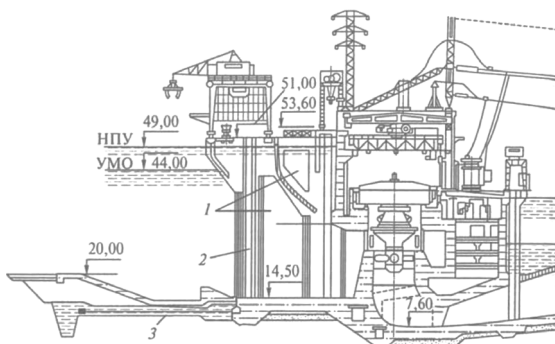
Рис. 1.45. Схема русловой ГЭС: 1 – прорези в быках; 2 – пазы в быках; 3 – анкерный понур
