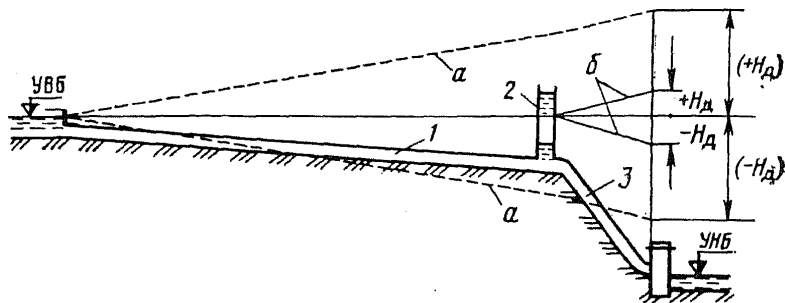
Рис. 1.33. Схема распространения максимального и минимального динамических давлений по длине трубопровода: а – при отсутствии уравнительного резервуара; б – при его наличии; 1 – деривационный трубопровод; 2 – уравнительный резервуар; 3 – турбинный трубопровод
