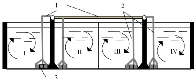
Рис. 2.2. Схема работы аэротенка: 1 – воздухопроводы; 2 – стояки; 3 – фильтросный канал; I, II, III, IV – коридоры
