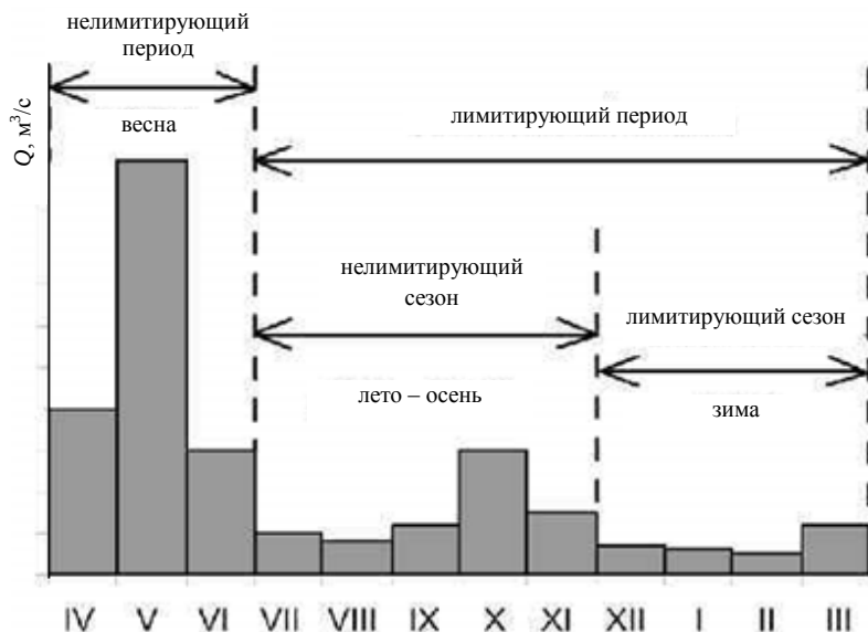
Рис. 3.3. Внутригодичное распределение стока
