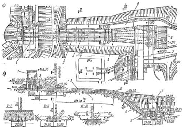
Рис. 1.43. Стационарный узел деривационной ГЭС с деривационным каналом: а – план стационарного узла; б – продольный разрез по оси турбинного трубопровода; 1 – здание водоприемника; 2 – турбинные трубопроводы железобетонные; 3 – то же, стальные открытые; 4 – температурные компенсаторы; 5 – анкерные опоры; 6 – турбинные трубопроводы стальные обетонированные и засыпанные щебнем; 7 – здание ГЭС; 8 – отводящий канал; 9 – аварийный отводящий канал
