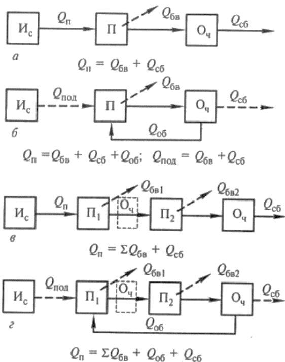
Рис. 1.6. Схемы использования воды в промышленности: а – прямоточная; б – оборотная; в – повторная; г – комбинированная; Q_{\text{п}} – полное водопотребление; Q_{\text{пол}} – подпитывание; Q_{\text{бв}} – безвозвратное водопотребление; Q_{\text{об}} – оборотные воды; Q_{\text{сб}} – воды, отводимые в водоем; I_{\text{с}} – источник воды; П, П 1 , П 2 – потребители воды; О ч – сооружения для отчистки вод
