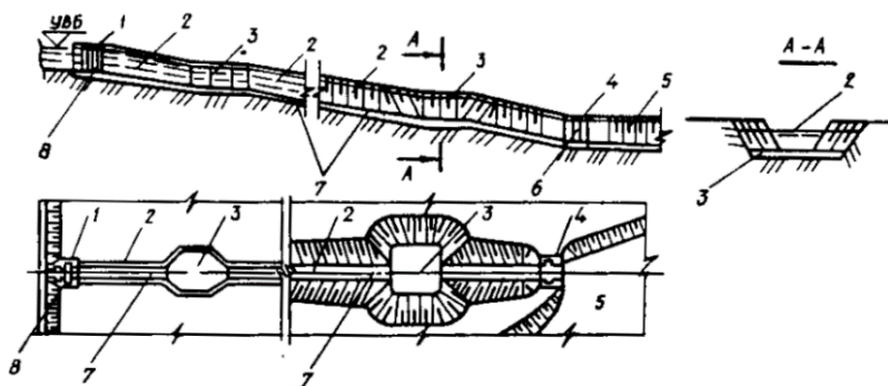
Рис. 1.15. Прудковый рыбоход:
