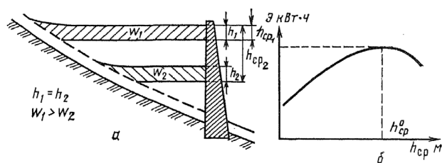
Рис. 2.7. Зависимость годовой выработки электроэнергии от глубины сработки водохранилища: a – схема сработки водохранилища; b – график зависимости объема выработки электроэнергии от величины сработки водохранилища
