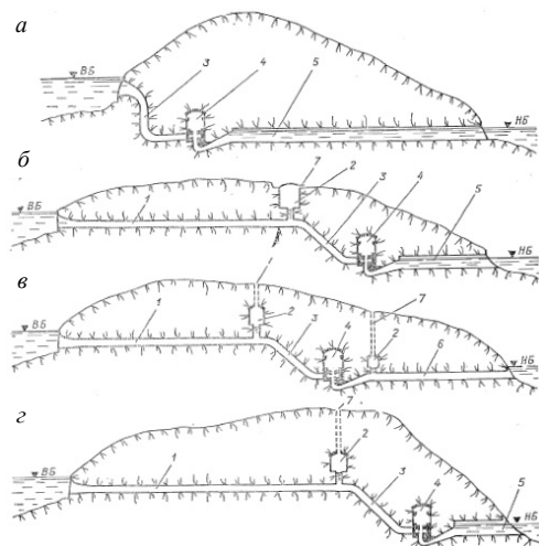
Рис. 1.44. Схема деривационных ГЭС с подземным размещением машинного зала: а-в – начало туннеля; б и в – в средней части туннеля; г – в конце туннеля; 1 – подводящий напорный туннель; 2 – уравнильный резервуар; 3 – турбинные водоводы; 4 – машинный зал; 5 – безнапорный отводящий туннель; 6 – напорный отводящий туннель; 7 – воздухопровод
