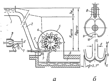
Рис. 1.28. Схема установки с активной (ковшовой) турбиной: а – схема установки; б – схема лопасти (ковша); 1 – напорный бассейн; 2 – турбинный трубопровод; 3 – сопло с регулирующей иглой; 4 – рабочее колесо; 5 – защитный кожух; 6 – отводящий канал; 7 – отклонитель струи; 8 – диск рабочего колеса; 9 – нож ковша; 10 – вырез в ковше для пропуска струи через ковш, находящийся в неблагоприятном положении к струе
