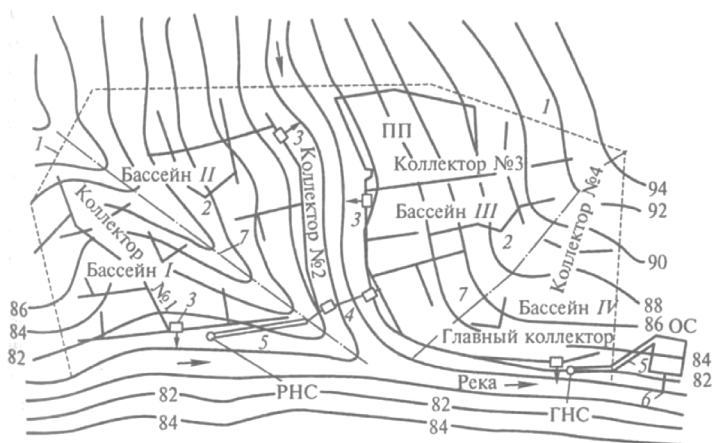
Рис. 1.3. Схема водоотведения: РНС – районная насосная станция; ГНС – главная насосная станция, ОС – очистные сооружения; ПП – промышленное предприятие; 1 – граница города; 2 – внешняя водоотводящая часть трубопровода; 3 – ливнеспуски; 4 – дюкер; 5 – напорные трубопроводы; 6 – выпуск очищенных сточных вод; 7 – линии водоразделов
