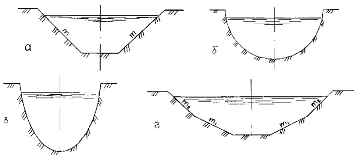
Рис. 1.7. Поперечные сечения мелиоративных каналов: а – трапецеидальное; б – круглое; в – параболическое; г – полигональное
