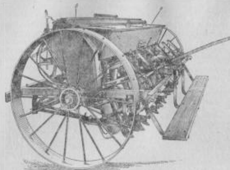
Рис. 61. Комбинированный свекловичный сеялка (а — шнек для семян, б — шнек для удобрений).
