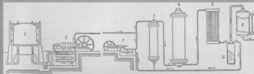
Рис. 16. Схема производства синтетического аммиака.
