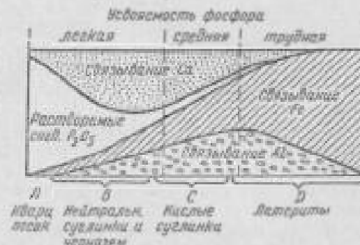
Рис. 25. Связывание фосфорной кислоты кальцием, железом и алюминием в разных почвах (схема).
