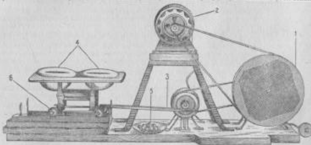
Рис. 3. Прибор для оценки физических свойств суперфосфата по методу Вискера.
