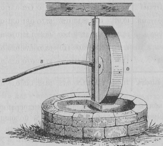
Рис. 68. Простая орѣхдробилка съ вертикальнымъ жерновомъ.
