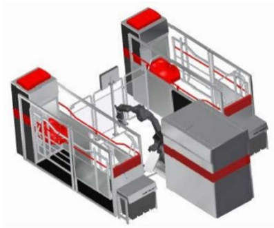
Рис. 6.8. Общий вид доильного робота Astrea фирмы «Insentec»
