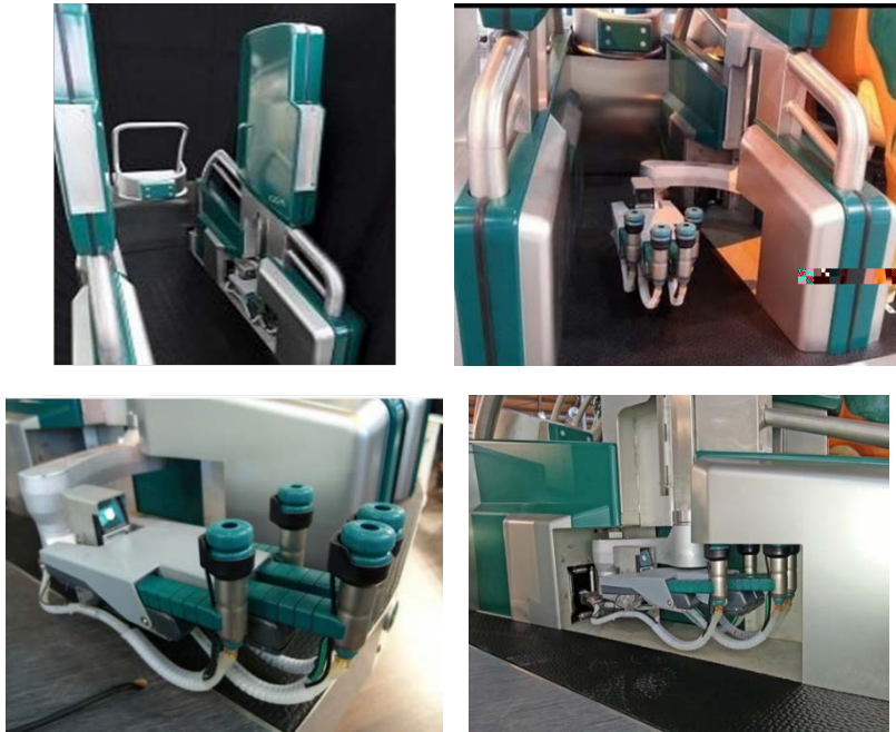
Рис. 6.13. Элементы автоматизированного доильного модуля Dairy ProQ
