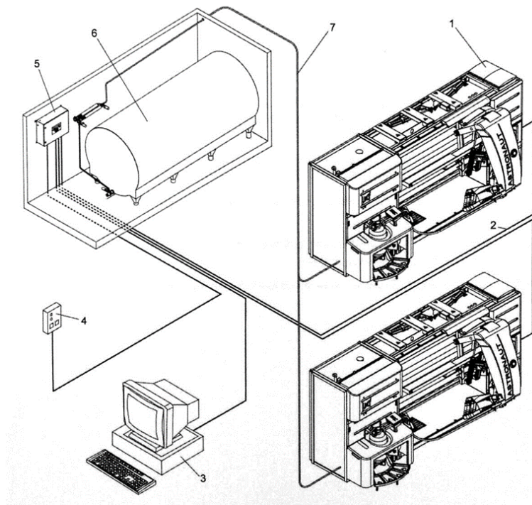
Рис. 6.4. Основные составляющие системы доения Astronaut: 1 – доильный робот; 2 – информационная сеть Т4С; 3 – персональный компьютер; 4 – сигнализатор; 5 – контроллер CRS+; 6 – танк-охладитель молока; 7 – молокопровод
