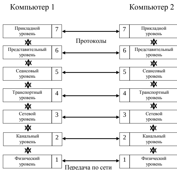
Рис. 3.2. Модель OSI
