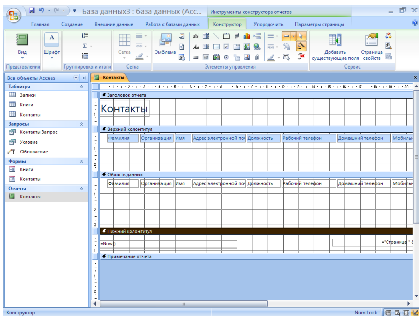
Рис. 4.52. Конструктор отчетов
