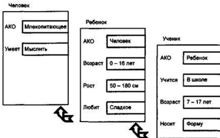
Рис. 5.5. Сеть фреймов
