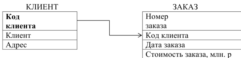
Рис. 4.3. Схема данных
