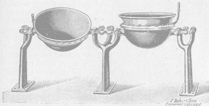
Рис. 3. Установка паровыхъ котловъ въ Англіи для варки варенья и желе. Котлы поднимаются вверхъ посредствомъ рычаговъ.
