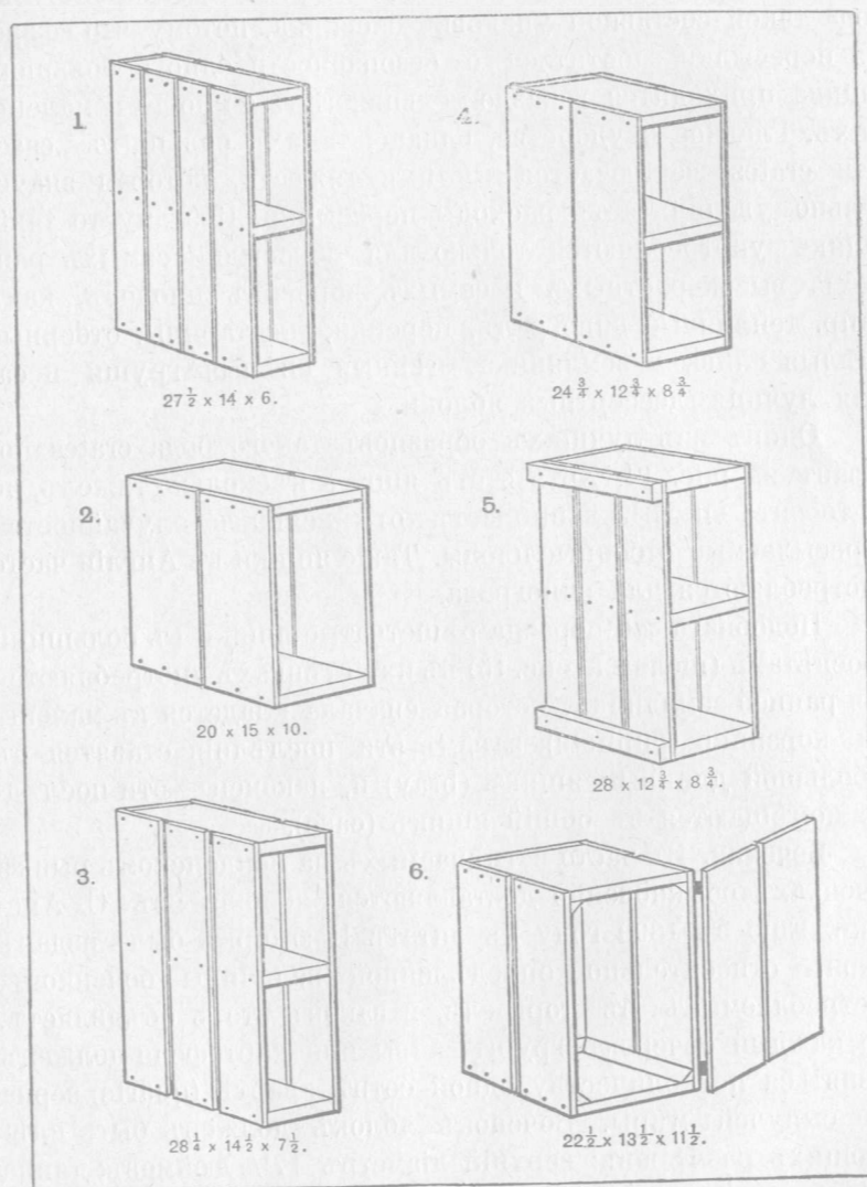
Рис. 11. Ящики для упаковки, встрѣчающіеся на англійскихъ рынкахъ. Размѣры показаны въ дюймахъ. Вмѣстимость ящика № 1—1856 кв. дюймовъ. № 2—2300 кв. дюймовъ. № 3—2457 кв. дюймовъ. № 4—2208 кв. дюймовъ. № 5—2496 кв. дюймовъ. № 6—2863 кв. дюймовъ. Цифры, поставленные внизу ящиковъ, обозначаютъ дюймы.
