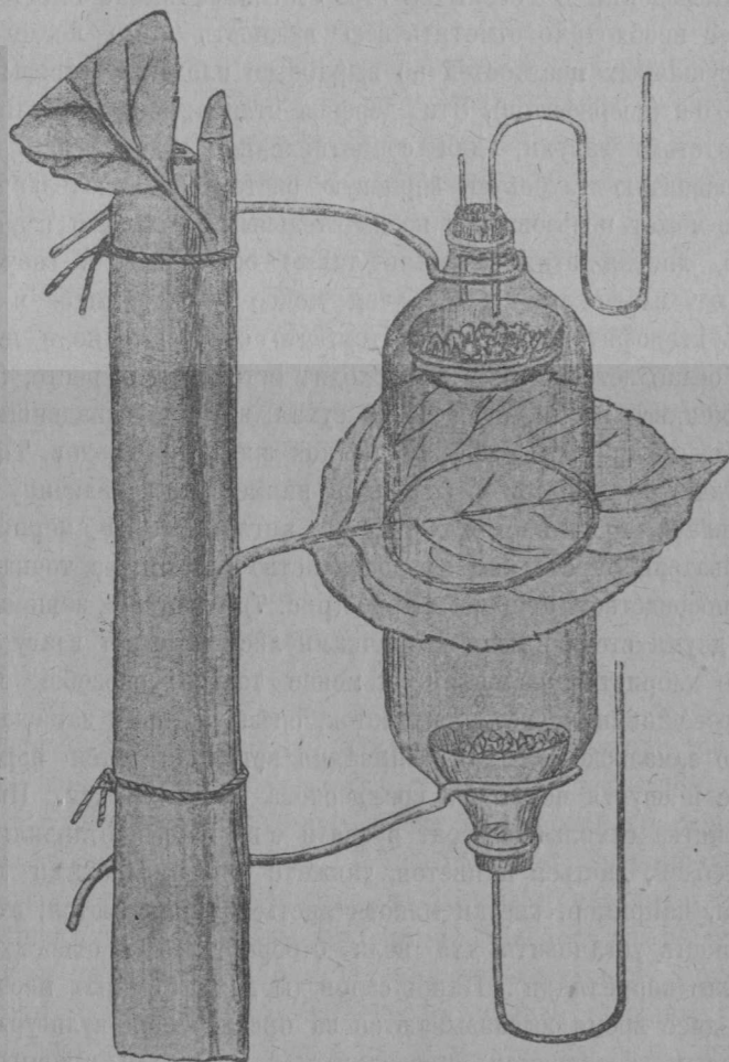
Рис. 7. Прибор Гарро для определения количества влаги, испаряемой верхнею и нижнею поверхностями листа. (Немн. уменьш.).
