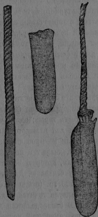
Рис. 11. Культурный фугас: слева—капсуля с фитилем, в середине—картушка, справа—готовый фугас, помещение в котором капсули изображено пунктиром.
