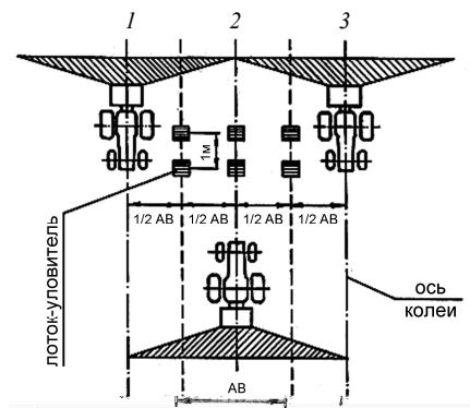
Рис. 9. Схема контрольной проверки доз внесения: 1, 2, 3 – номер прохода агрегата; АВ – рабочая ширина захвата
