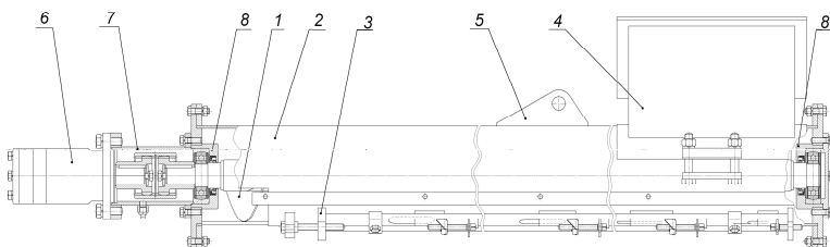
Рис. 7. Штанга: 1 – шнек; 2 – кожух; 3 – регулировочное устройство; 4 – загрузочная горловина; 5 – зацеп; 6 – гидромотор; 7 – муфта; 8 – подшипниковый узел
