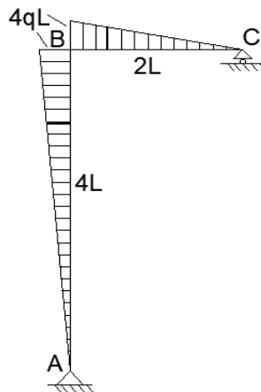
Рис. 13. Единичная эпюра моментов
