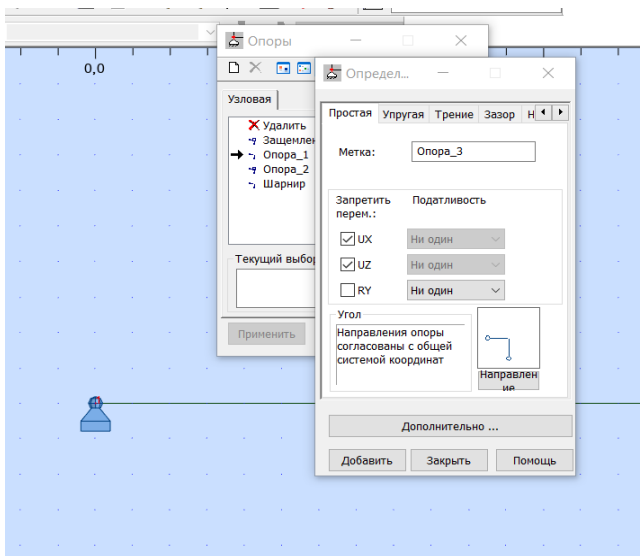
Рис. 3. Создание опор балки
