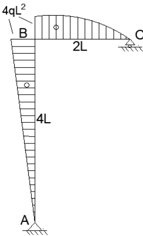
Рис. 12. Грузовая эпюра моментов
