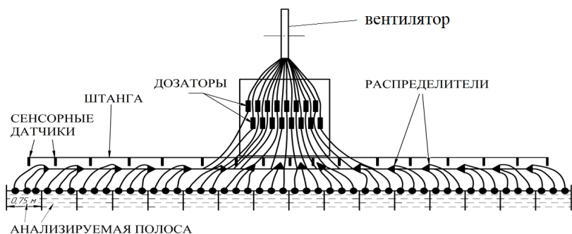
Рис. 14. Принципиальная схема пневматической высевальной системы для дифференцированного внесения гранулированных минеральных удобрений
