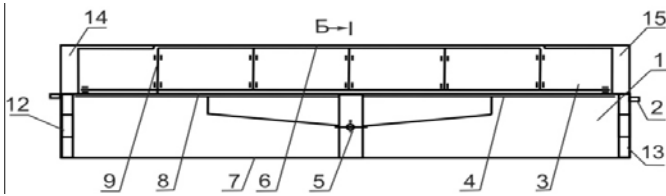
Рис. 3. Горизонтальный разрез самокормушки для свиней
