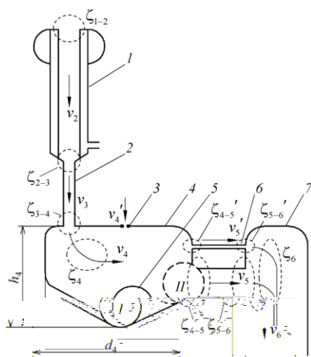
Рис. 1. Конструктивно-технологическая схема доильного аппарата с четырехкамерным коллектором:
