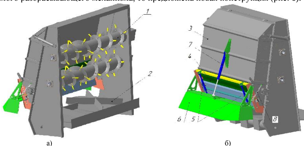
Рис. 6. Схема комбинированного рабочего органа для внесения мелиорантов: а) вид сзади; б) вид спереди;
