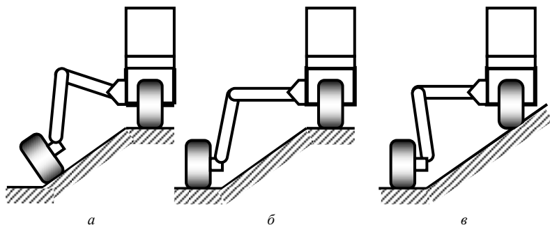
Рис. 2.58. Схема вариантов зон передвижения трехопорного каналоочистителя: а – берма и откос; б – берма и дно; в – откос и дно
