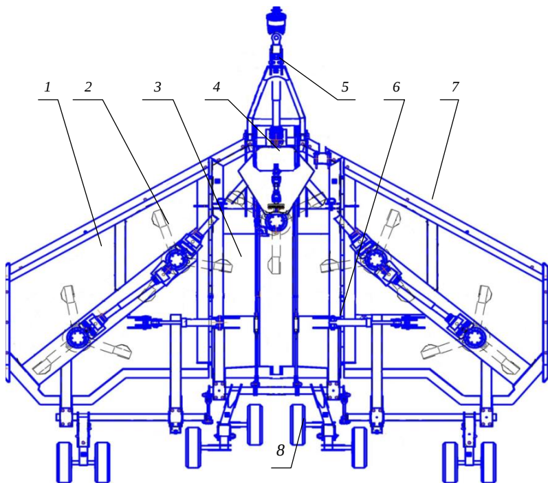
Рис. 5.10. Конструктивная схема косилки КП-6,2:
