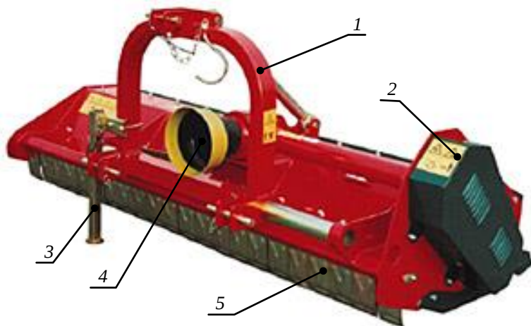
Рис. 5.4. Общий вид косилки-измельчителя VN Master Cut TSA: 1 – навесное устройство; 2 – редуктор привода барабана; 3 – сница; 4 – узел присоединения привода косилки к BOM; 5 – измельчающий аппарат
