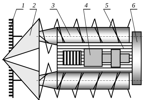
Рис. 4.79. Косилка КП-2,0 на шнековых понтонах: 1 – рабочий орган; 2 – отвал; 3 – шнековые понтоны; 4 – силовая установка; 5 – палуба; 6 – редуктор
