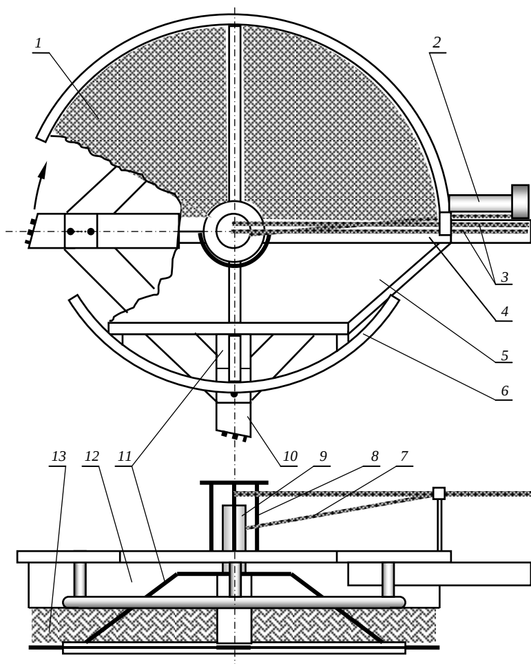
Рис. 4.22. Схема одноаторной четырехножевой косилки КР-1,3: 1 – верхняя часть кожуха; 2 – гидроцилиндр; 3 – шланги; 4 – рукоять; 5 – верхняя часть кожуха; 6 – защитная дуга; 7 – дренажный шланг; 8 – ограждение; 9 – гидромотор; 10 – зубчатые ножи; 11 – ротор; 12 – задняя часть кожуха; 13 – цепной фартук
