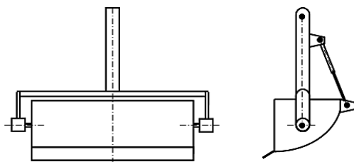
Рис. 2.45. Схема поворотного ковша с вилообразной рукоятью
