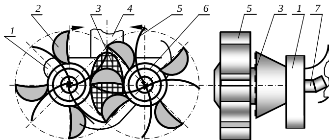
Рис. 8.18. Схема двухроторного черпакового разрыхлителя: 1 – редуктор; 2 – черпаки; 3 – заборная сетка; 4 – всасывающая труба; 5 – очистители; 6 – ступицы; 7 – гидропривод
