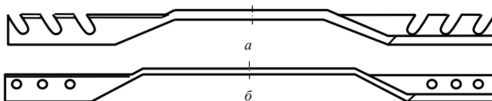
Рис. 5.13. Ножи газонокосилок с плоскостями для подъема срезанной травы и с наклонными прорезями ( a ) и отверстиями ( б ) в этих плоскостях: a – нож фирмы Gator; б – нож фирмы Stens
