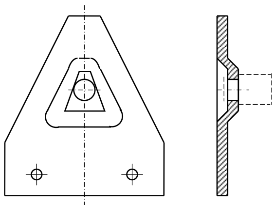
Рис. 4.14. Схема ножа косилки с двухножевым режущим аппаратом
