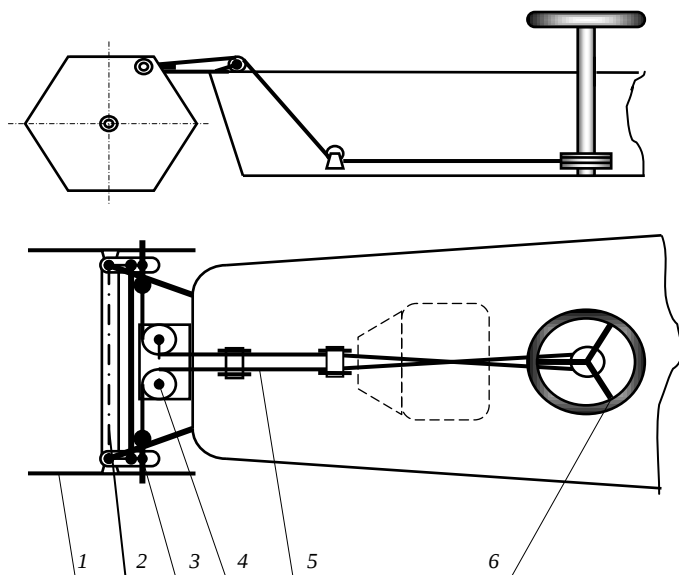
Рис. 4.72. Схема рулевого управления косилки ЛК-12: 1 – рули; 2 – поперечина; 3 – регулировочные тяги; 4 – блоки; 5 – тросовые тяги; 6 – рулевое колесо
