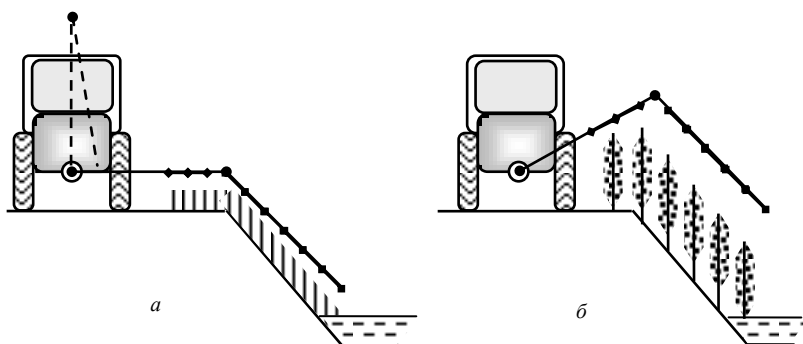
Рис. 4.90. Основные положения штангового опрыскивателя: а – транспортное и при обработке низкорослой растительности; б – при обработке высокорослой растительности
