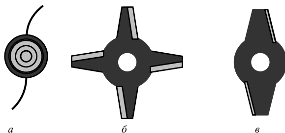
Рис. 4.59. Типы сменных роторов ручных косилок: а – с лесками; б – дисковый четырехконсольный; в – дисковый двухконсольный
