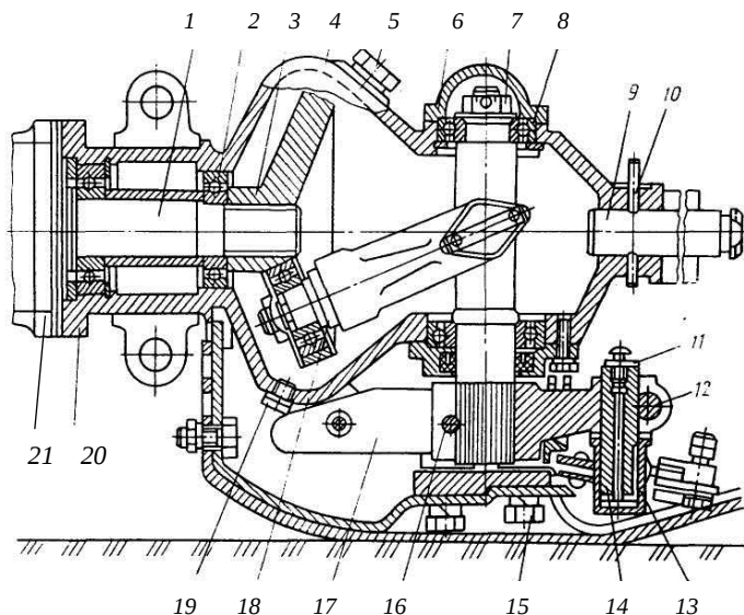
Рис. 4.6. Конструкция привода с вилкой и кривошипом сегментного аппарата:
