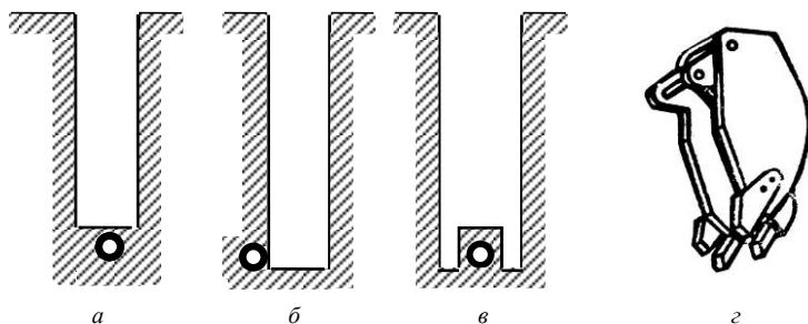
Рис. 6.1. Схемы вскрытия дрены:
