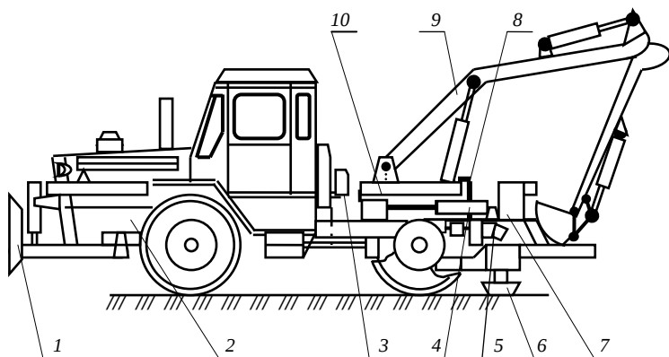
Рис. 3.4. Ремонтно-эксплуатационный агрегат АРЭ: 1 – бульдозерное оборудование; 2 – базовый трактор; 3 – гидрораспределитель; 4 – гидроцилиндр; 5 – насос; 6 – опоры; 7 – бак гидросистемы; 8 – стопор; 9 – стрела; 10 – поворотная платформа
