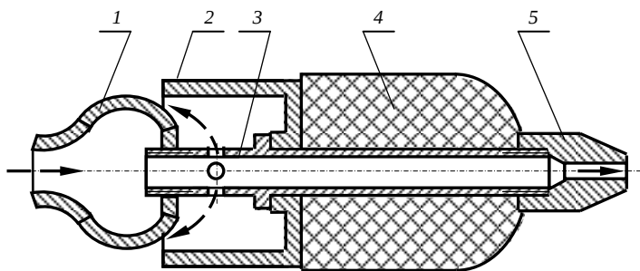
Рис. 7.8. Гидрореактивный снаряд:
