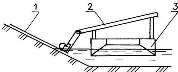
Рис. 4.76. Плавающая косилка с боковым сегментным рабочим органом: 1 – рабочий орган; 2 – рама; 3 – мотобот
