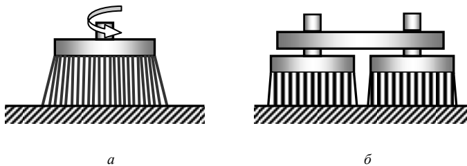
Рис. 2.27. Схема щетки-фрезы с осью вращения, перпендикулярной обрабатываемой поверхности: а – щетка с одним рабочим элементом; б – с двумя элементами
