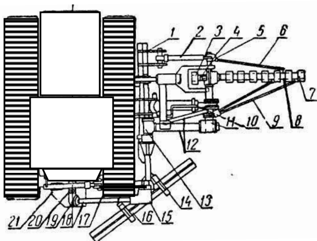
Рис. 2.7. Каналоочиститель со скребковым рабочим органом: 1 – рама; 2, 10, 21 – гидроцилиндры; 3 – скребки; 4 – ведущая звездочка; 5, 12, 18, 20 – валы; 6, 9 – растяжки; 7 – натяжной ролик; 8 – рама рабочего органа; 11, 13, 15, 19 – редукторы; 14 – гидроцилиндры; 16 – кавальероразравниватель; 17 – базовая машина
