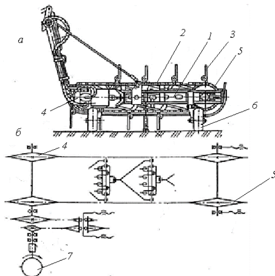
Рис. 4.60. Конвейерный цепной подборщик:
