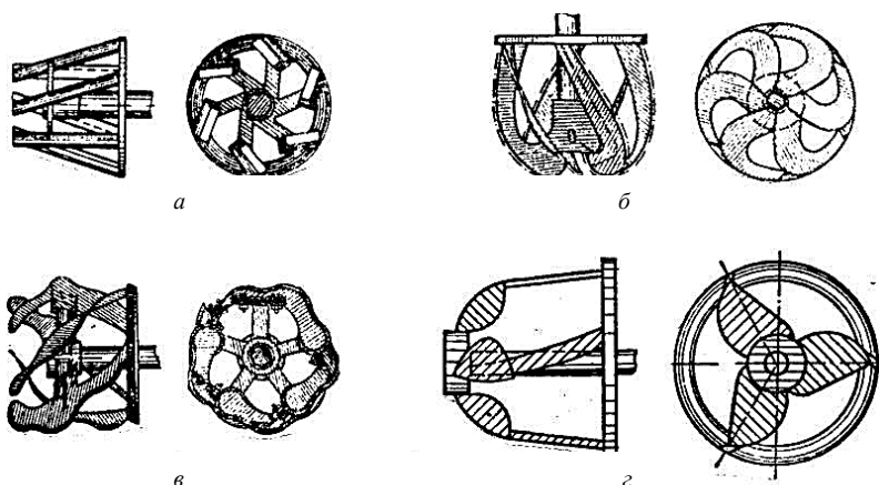
Рис. 8.14. Фрезы наиболее типичных конструкций: а – открытая с плоскими ножами; б – закрытая (митрообразная) с ножами двойной кривизны; в – полуоткрытая с ножами волнообразной формы; г – с отвальными-режущими лопастями
