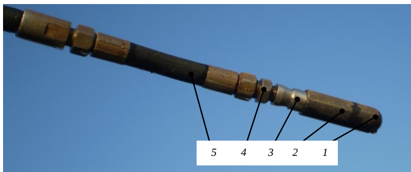
Рис. 6.35. Дренопромывочная головка машины УПД-120, оснащенная излучателем сигнала:
