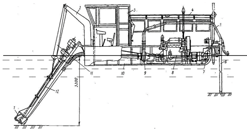
Рис. 8.2. Схема малогабаритного земснаряда:
