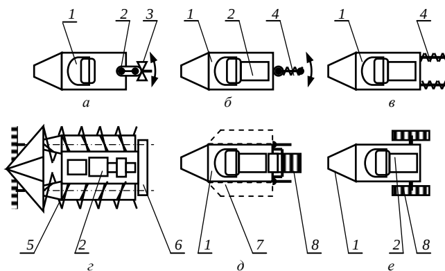
Рис. 4.65. Схемы плавучих косилок:
