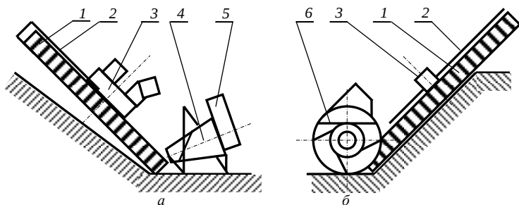
Рис. 2.33. Схема комбинированных рабочих органов:
