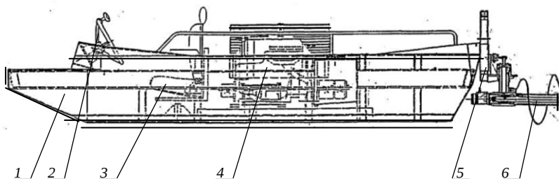
Рис. 4.66. Мотобот с поворотным шнековым винтом:
