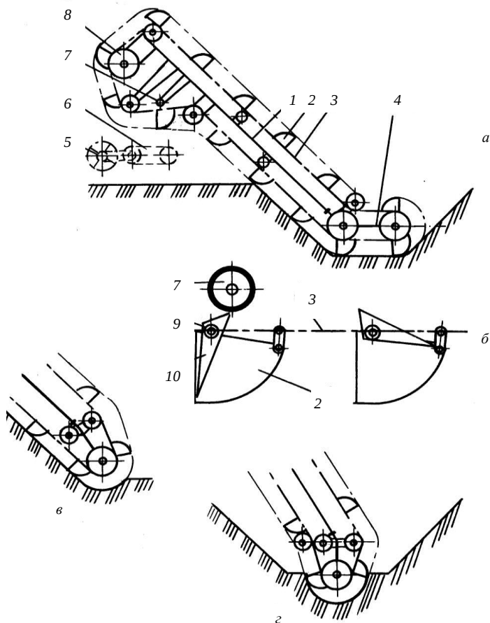
Рис. 2.1. Схема многоковшового цепного рабочего органа поперечного копания: а – рабочий орган в сборе; б – процесс выгрузки грунта; в – схема очистки откоса; з – схема очистки дна;
