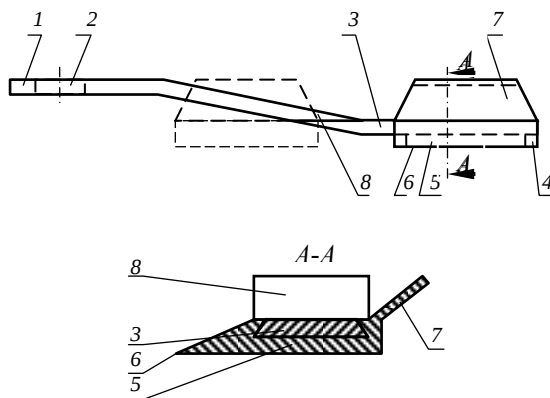
Рис. 5.15. Нож косилки-измельчителя со съемной режущей частью:
