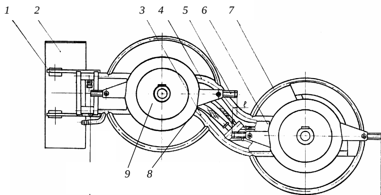
Рис. 4.29. Двухроторный рабочий орган: 1 – проушины; 2 – узел присоединения; 3, 4 – маслопроводы; 5 – ножи; 6 – корпус; 7 – тарельчатые опоры; 8 – крестовина; 9 – колпаки
