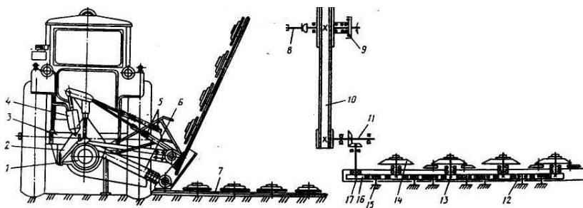
Рис. 4.34. Четырехроторная косилка на базе колесного трактора:
