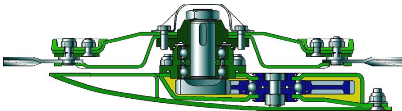
Рис. 4.41. Поперечный разрез по оси ротора косилок фирм Claas и Krone
