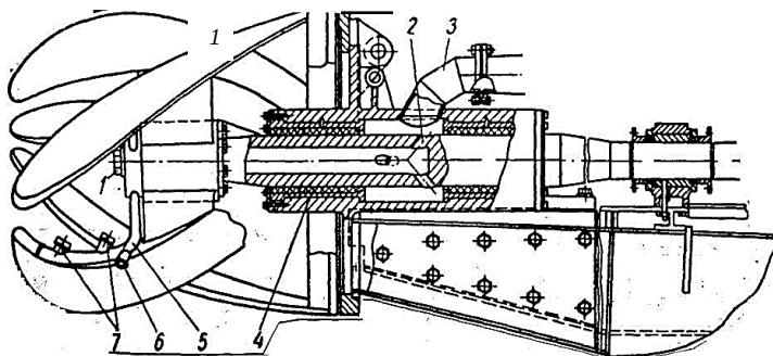
Рис. 8.21. Фрезерно-гидравлический разрыхлитель: 1 – лобовой насадок; 2 – каналы; 3 – водопровод; 4 – головной подшипник; 5 – подающие патрубки; 6 – боковые разрыхляющие насадки; 7 – смазывающе-подводящие насадки
