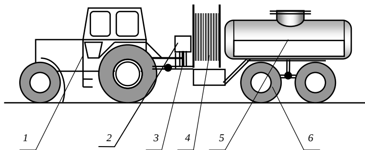
Рис. 6.23. Компоновочная схема дрепопромывочной машины ДП-10А:
