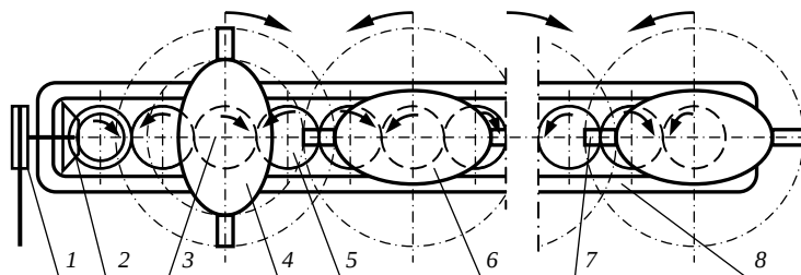
Рис. 4.36. Кинематическая схема многороторного рабочего органа: 1 – ременной привод; 2 – конический редуктор; 3 – ведущие шестерни; 4, 6 – диски; 5 – промежуточные шестерни; 7 – ножи; 8 – корпус
