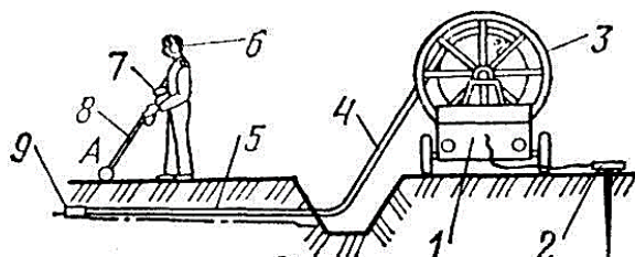
Рис. 6.33. Схема диагностирования дренажной системы с помощью трассоискателя:
