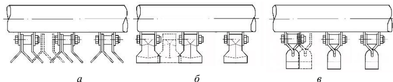
Рис. 5.3. Типы ножей косилки КИ-3:
