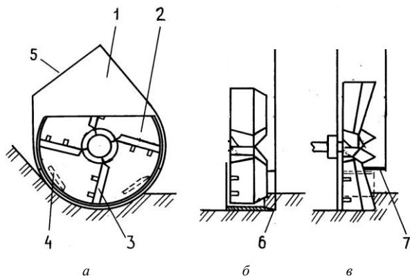
Рис. 2.15. Схемы фрезерных рабочих органов с осью вращения, параллельной оси канала: а – вид спереди; б – вид сбоку фрезы с кожухом, опирающимся о дно; в – вид сбоку фрезы с кожухом, не опирающимся о дно; 1 – кожух; 2 – диск; 3 – ножи-лопатки; 4 – дополнительные ножи; 5 – выбросное окно; 6 – режущая кромка; 7 – противорежущая кромка
