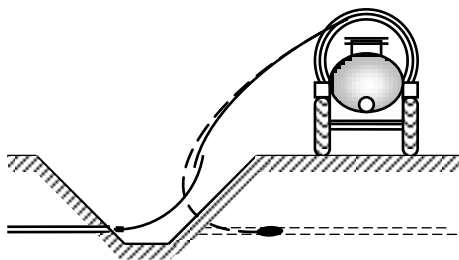
Рис. 6.22. Схема расположения дрепоочистителя по отношению к каналу
