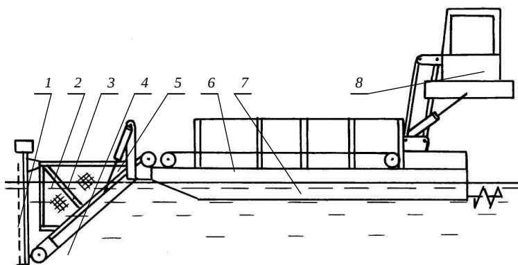
Рис. 4.85. Схема плавучего комбайна для удаления водной растительности: 1 – U-образный режущий аппарат; 2 – П-образная рама; 3 – сетчатые щиты; 4 – пластинчатый транспортер; 5 – гидравлическое управление; 6 – движущееся дно; 7 – бункер; 8 – кабина
