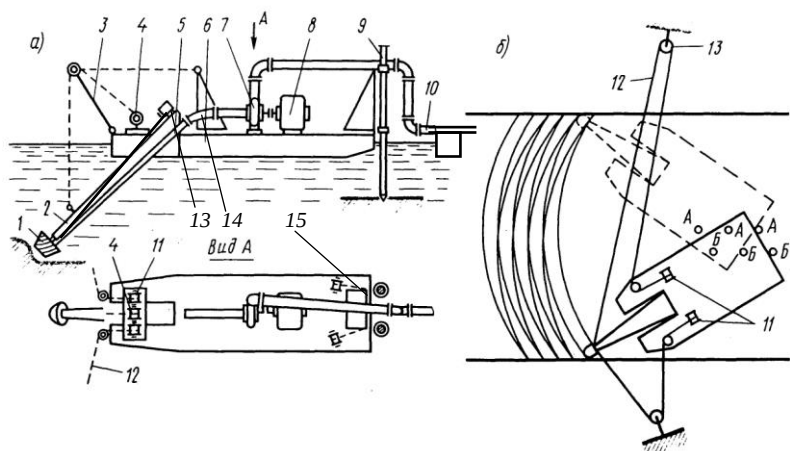
Рис. 8.1. Схема земснаряда:
