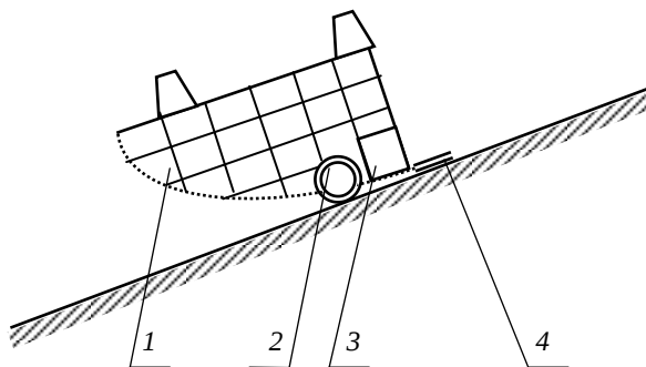
Рис. 4.56. Схема рабочего органа корзины-косилки: 1 – ковш; 2 – опорные колеса; 3 – привод; 4 – режущий аппарат
