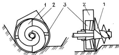
Рис. 2.30. Шнекороторный рабочий орган: 1 – конический шнек; 2 – кожух; 3 – метатель
