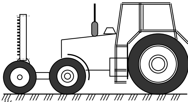
Рис. 2.56. Вариант каналаочистителя с дополнительной передней колесной опорой
