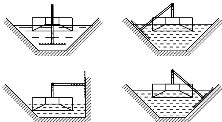
Рис. 4.74. Основные положения рабочего органа косилки с поворотным Т-образным рабочим органом
