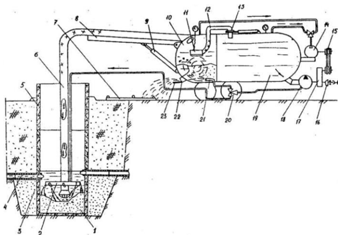
Рис. 7.3. Схема работы МОК-10:
