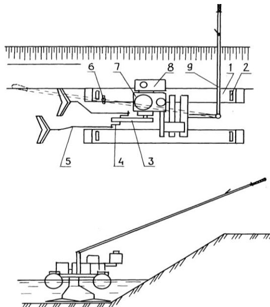
Рис. 4.64. Переносная плавучая косилка: 1 – цилиндрические понтоны; 2 – рукоятки; 3 – передача; 4 – кривошипы; 5 – тяги со стреловидными ножами; 6 – стойка; 7 – двигатель; 8 – топливный бак; 9 – штанга
