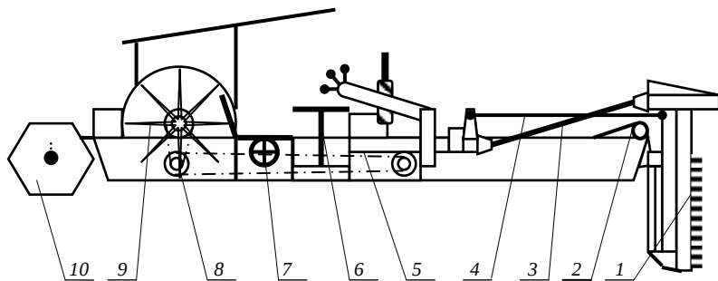
Рис. 4.71. Схема лодки-косилки ЛК-12: 1 – Т-образный режущий аппарат; 2 – трос; 3 – карданная передача; 4 – рама; 5 – двигатель; 6 – рулевое колесо; 7 – лебедка; 8 – цепная передача; 9 – гребные колеса; 10 – рули
