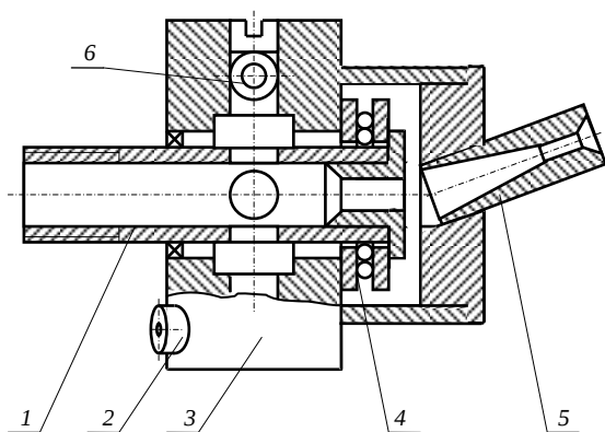
Рис. 6.17. Головка с вращающимся корпусом:
