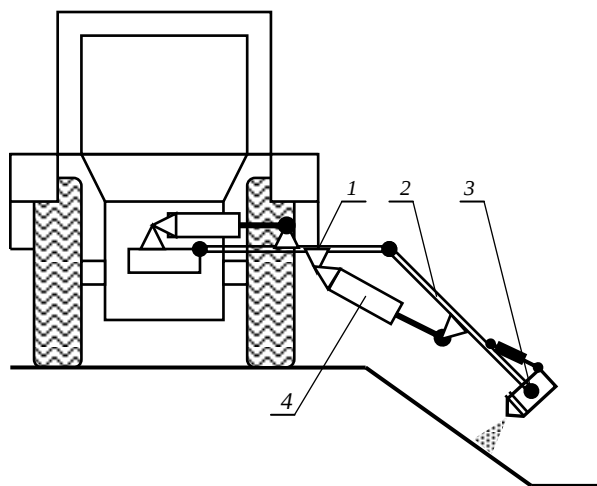
Рис. 4.89. Схема машины огневого действия: 1 – стрела; 2 – рукоять; 3 – форсунка; 4 – гидроуправление
