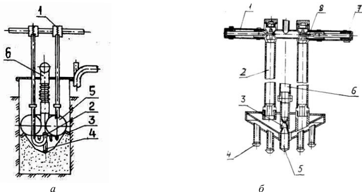
Рис. 7.4. Ручные устройства для механизации работ: а – при очистке колодцев; б – при очистке каналов; 1, 7 – рукоятки; 2 – эжектор; 3 – насадки; 4 – сопла; 5 – торообразная камера; 6 – пульпопровод; 8 – клапан
