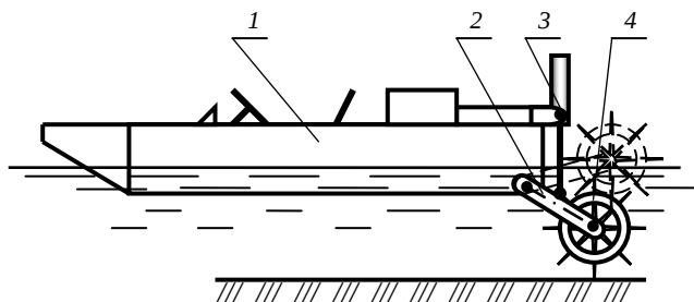
Рис. 4.78. Косилка для мелководья: 1 – моторбот; 2 – цепная передача; 3 – гидроцилиндр; 4 – гребные колеса
