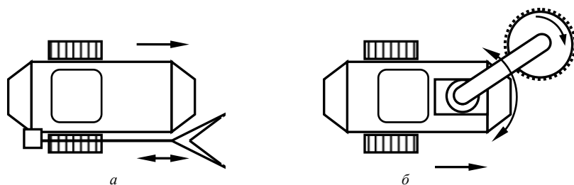
Рис. 4.67. Схемы косилок: а – с V-образным рабочим органом; б – с дисковой пилой
