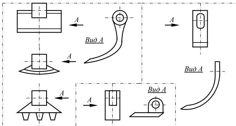
Рис. 4.50. Ножи косилки-измельчителя с шарнирно закрепленными Г-образными ножами
