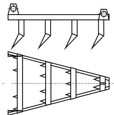
Рис. 2.43. Корчущая борона
