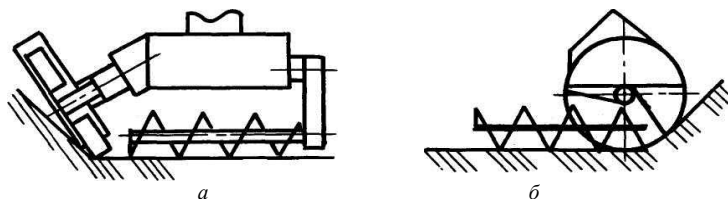
Рис. 2.10. Шнековые цилиндрические рабочие органы с осью вращения, параллельной дну канала: а – совмещенный с фрезой (торцевая центральная подача); б – с лопастным метателем
