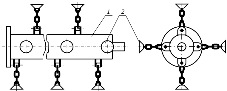
Рис. 4.49. Схема ротора косилки-измельчителя с шарнирно закрепленными чашечными ножами: 1 – барабан; 2 – ножи
