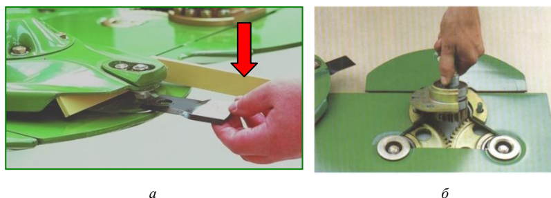
Рис. 4.43. Приемы переналадки косилок фирм Claas и Krone: а – замена ножа; б – переустановка ведомой шестерни ротора
