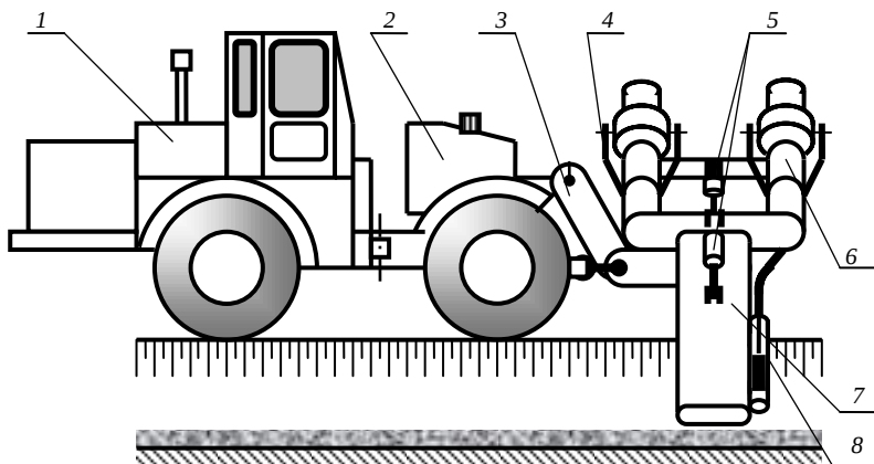
Рис. 2.29. Схема газодинамического (газоструйного) каналаочистителя: 1 – базовый трактор; 2 – топливный бак; 3 – навеска; 4 – рама; 5 – гидроцилиндры; 6 – реактивные авиационные двигатели; 7 – газопровод; 8 – горелка
