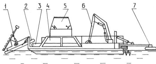
Рис. 4.86. Схема плавучего комбайна с колесными опорами: 1 – режущий аппарат; 2, 3 – транспортирующие органы; 4 – бункер; 5 – кабина; 6 – грейферное оборудование; 7 – колесные опоры
