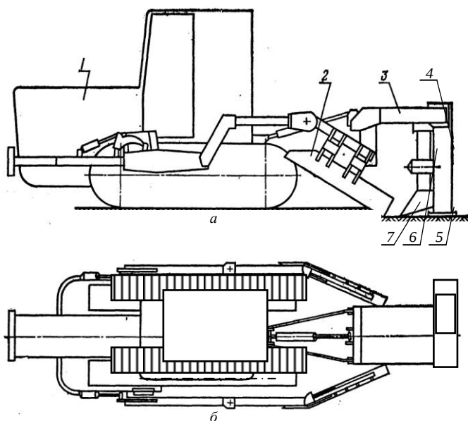
Рис. 2.37. Схема отвально-фрезерного каналочистителя:
