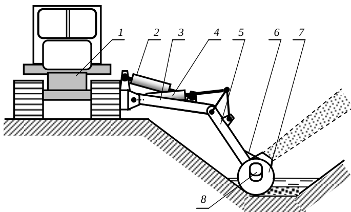
Рис. 2.14. Схема работы каналоочистителя с фрезерным рабочим органом: 1 – трактор; 2, 4 – гидроцилиндры; 3 – рама; 5 – рукоятка; 6 – тяга; 7 – рабочий орган; 8 – гидромотор
