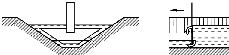
Рис. 2.25. Схема гидравлического рыхления наносов посредством заслонки
