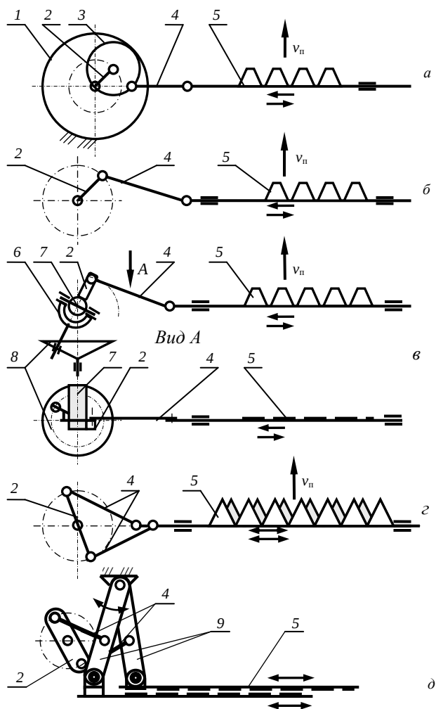
Рис. 4.5. Кинематические схемы сегментных режущих аппаратов: a – сегментного с планетарным приводом; б – сегментного с кривошипным приводом; в – сегментного с вилкой и кривошипом; г – сегментного двухножевого с кривошипным приводом; д – сегментного двухножевого с кривошипно-кулисным приводом; 1 – корончатое колесо; 2 – кривошип; 3 – сателлит; 4 – шатун; 5 – сегменты; 6 – вал вилки; 7 – вал; 8 – диск; 9 – кулисы
