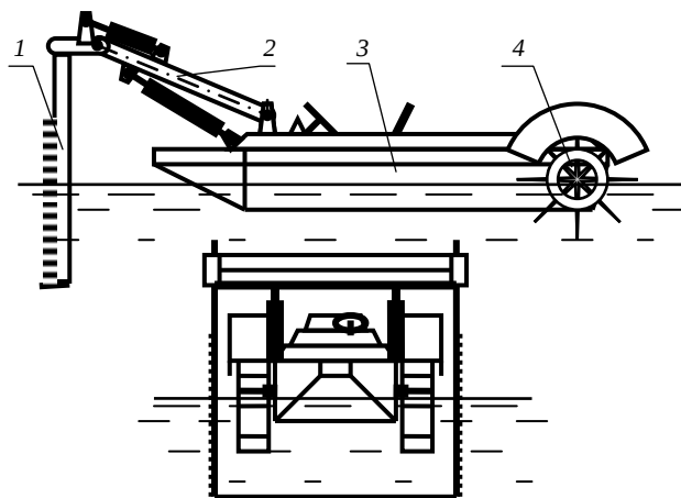
Рис. 4.77. Схема косилки с П-образным рабочим органом: 1 – рабочий орган; 2 – П-образная рама; 3 – моторбот; 4 – гребные колеса
