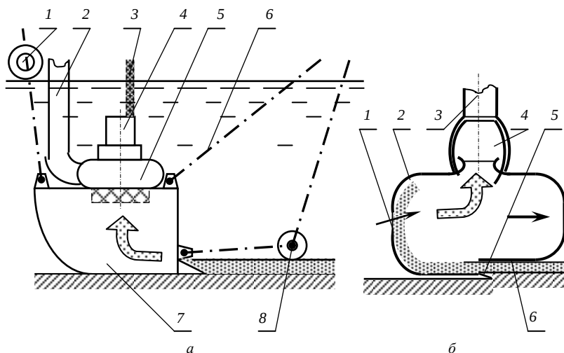
Рис. 8.23. Одноковшовые рабочие органы:
