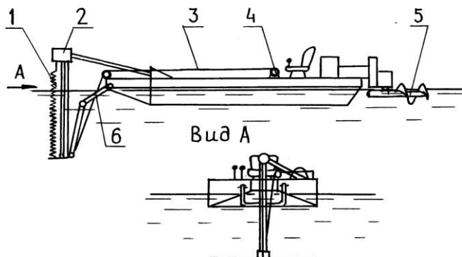
Рис. 4.69. Схема косилки с Т-образным рабочим органом: 1 – Т-образный рабочий орган; 2 – редуктор; 3 – канат; 4 – лебедка; 5 – шнековый винт; 6 – двухзвенная стрела
