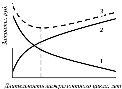
Рис. 1.1. Зависимость затрат от периодичности КР:
