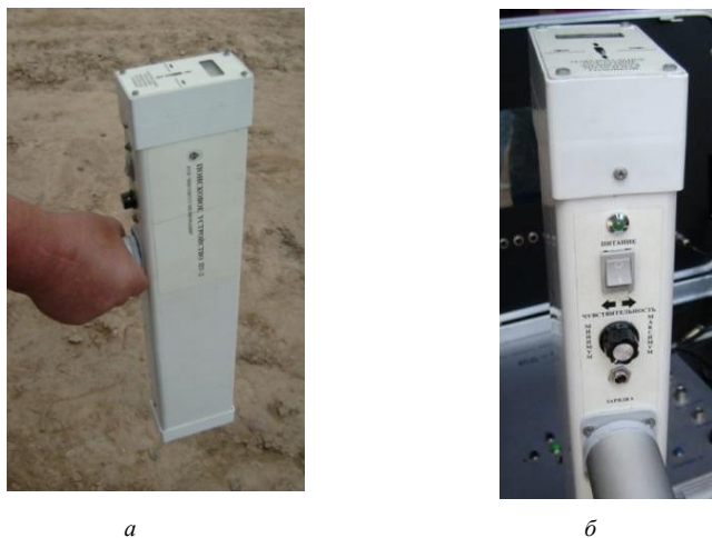
Рис. 6.42. Поисковое устройство ПУ-2: а – общий вид; б – передняя панель
