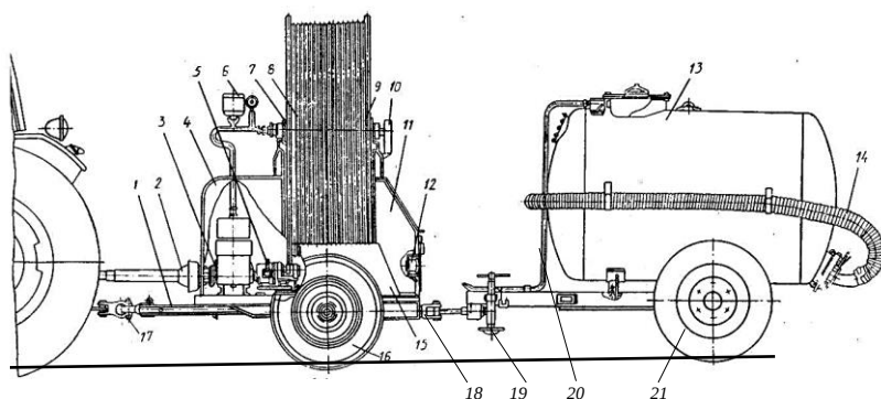
Рис. 6.21. Дренопромывочная машина МР-18:
