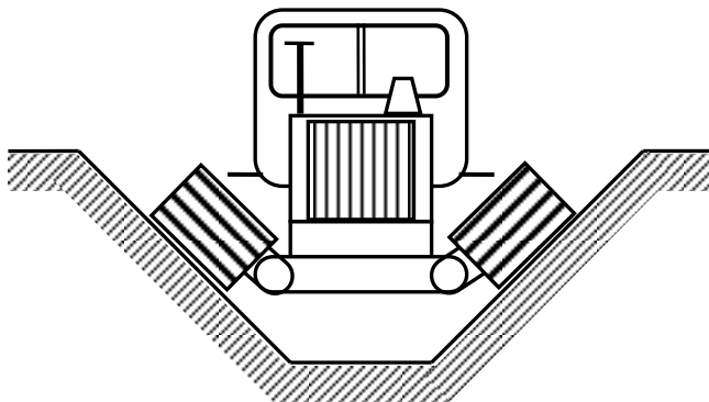
Рис. 2.63. Схема гусеничного внутриканального каналочистителя с наклоняемыми гусеницами
