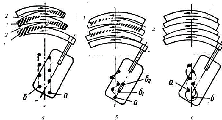
Рис. 8.8. Схема рабочих ходов земснаряда: а – с фиксированной установкой свай; б – со сваями, перемещающимися в прорези по продольной оси земснаряда; в – с роторным свайным аппаратом; 1 – зоны на которых грунт был забран; 2 – зоны пропуска грунта
