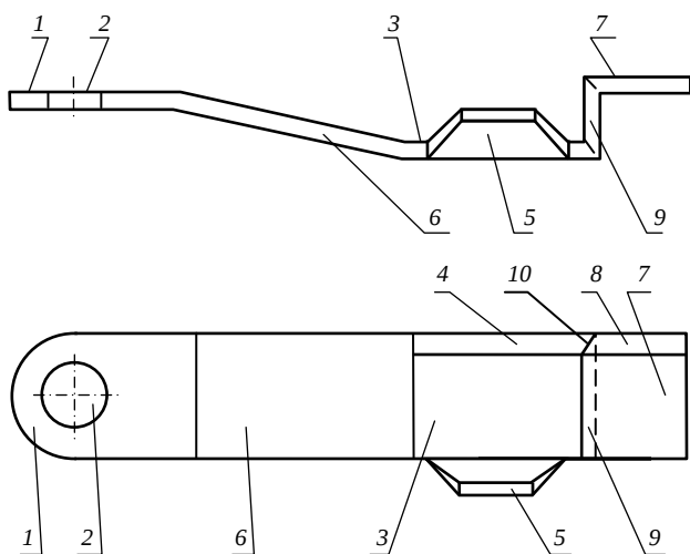
Рис. 5.16. Изогнутый нож косилки-измельчителя:
