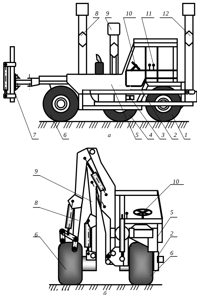
Рис. 2.57. Схема трехопорного каналаочистителя АСМ: a – вид слева; б – вид спереди; 1, 6 – основные опоры; 2 – рама; 3 – насос; 4 – вспомогательная опора; 5 – силовая установка; 7 – переднее навесное устройство; 8 – боковое навесное устройство; 9 – рабочее оборудование; 10, 11 – органы управления; 12 – заднее навесное устройство
