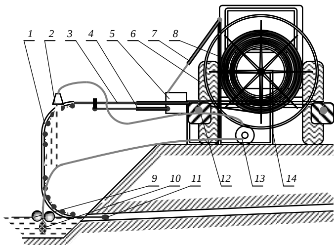
Рис. 6.25. Навесное дренапромывочное оборудование Professional:
