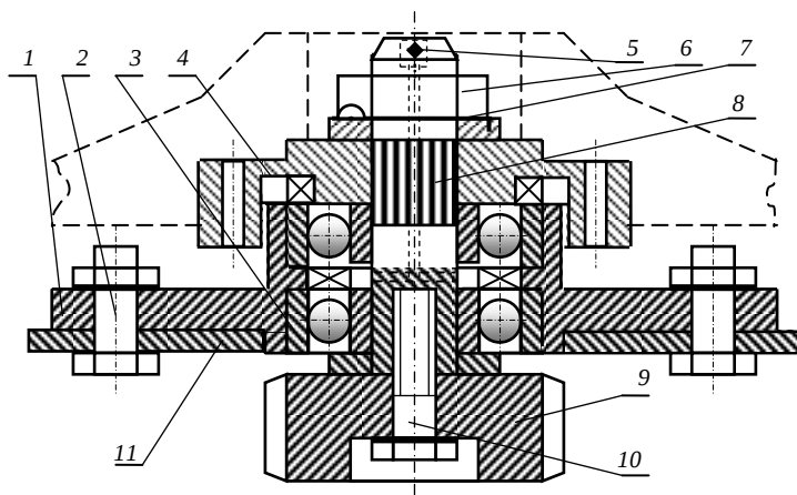
Рис. 4.40. Схема привода роторов рабочего органа многороторной косилки: 1 – стакан; 2 – болты; 3 – подшипники; 4 – фланец; 5 – пресс-масленка; 6 – гайка; 7 – шайба; 8 – вал ротора; 9 – приводная шестерня; 10 – болт; 11 – верхняя часть корпуса редуктора
