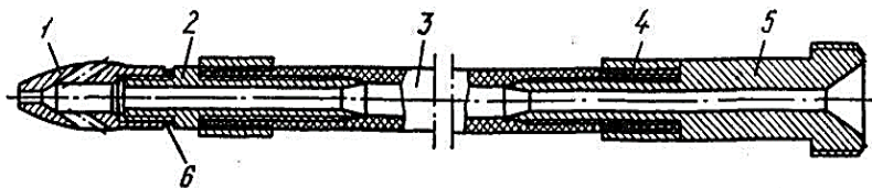
Рис. 6.12. Конструкция шланга с головкой: 1 – головка; 2, 5 – штуцеры; 3 – шланг; 4 – кольцо; 6 – прокладка
