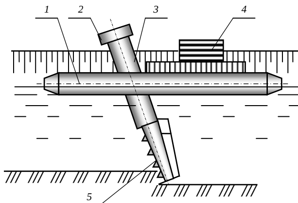
Рис. 2.12. Схема плавучего каналоочистителя:
