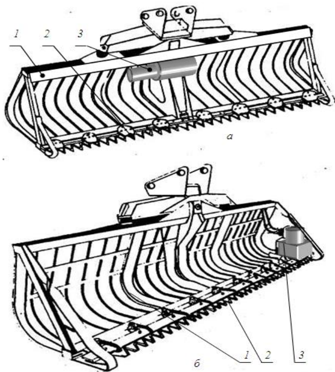
Рис. 4.55. Рабочий орган ковша-косилки: а – с центральным расположением привода; б – с боковым; 1 – ковш; 2 – режущий аппарат; 3 – гидромотор с редуктором
