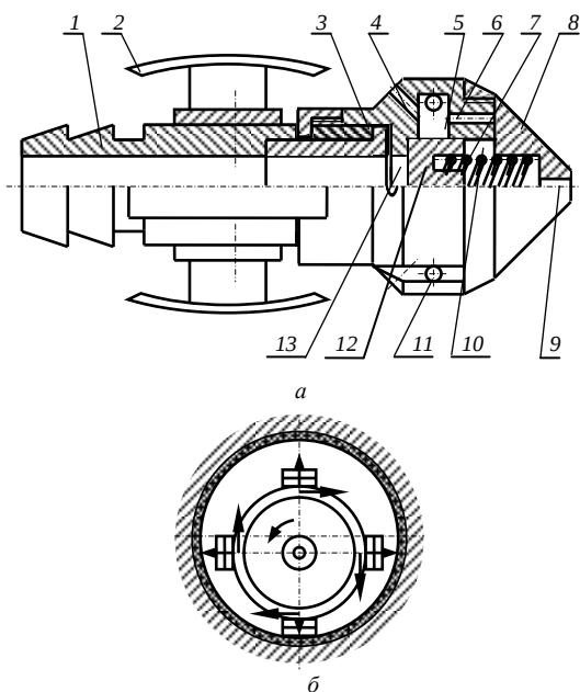
Рис. 6.19. Головка с импульсной подачей воды: а – вид сбоку; б – расположение головки в дрене; 1 – штуцер корпуса; 2 – направляющие лыжи; 3 – подшипник скольжения; 4 – выходные задние отверстия; 5, 10, 13 – камеры; 6 – продольные каналы; 7 – пружина; 8 – вращающаяся головка; 9 – переднее отверстие; 11 – тангенциальные отверстия; 12 – поршень
