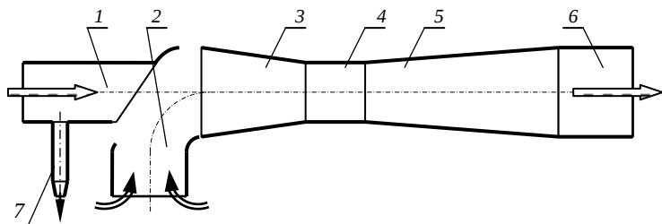
Рис. 7.7. Грунтосос:
