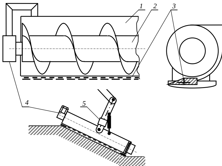
Рис. 4.54. Рабочий орган шнека-косилки: 1 – кожух; 2 – шнек; 3 – сегментно-пальцевый режущий аппарат; 4 – гидромотор; 5 – амортизирующий узел
