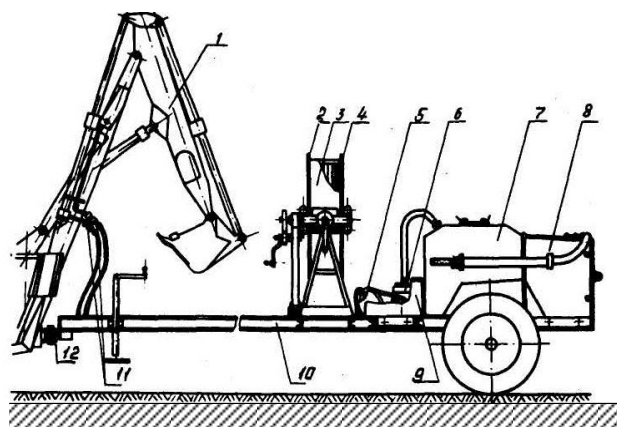
Рис. 6.30. Ремонтный комплекс К-68А:
