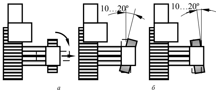
Рис. 2.61. Схема изменения расстояния между гусеницами каналаочистителя МР-15: а – изменение колеи при неподвижном экскаваторе; б – изменение колеи в движении
