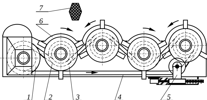
Рис. 4.45. Кинематическая схема рабочего органа косилки с ременным приводом роторов:
