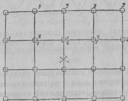
Рис. 15. Квадратная планировка. Пересекающиеся дуги показывают точку перпендикуляра. Цифрами обозначены колышки: 1 и 3 — крайн., 2 — средн.
