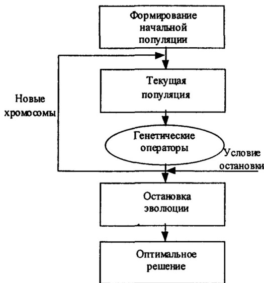
Рис. 9.2. Генетический алгоритм
