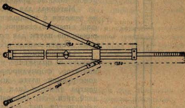
Черт. 17. Измеритель ширины борозд автора статьи.
