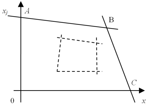
Рис. 19. Область допустимых решений задачи линейного программирования – выпуклая область OABC
