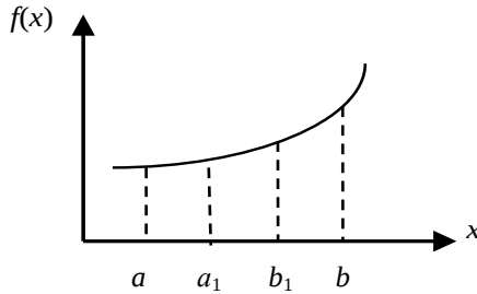
Рис. 14. Точка минимума должна быть в отрезке [a, b]
