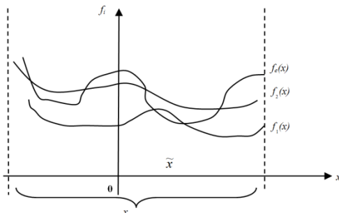
Рис. 23. Первый вариант решения задачи векторной оптимизации
