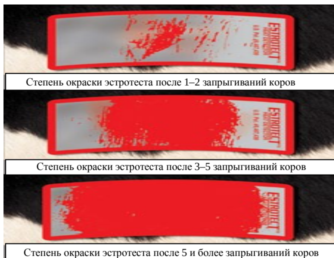
Рис. 6.6. Изменение степени окраски эстротестов в зависимости от числа запрыгиваний на корову в период половой охоты
