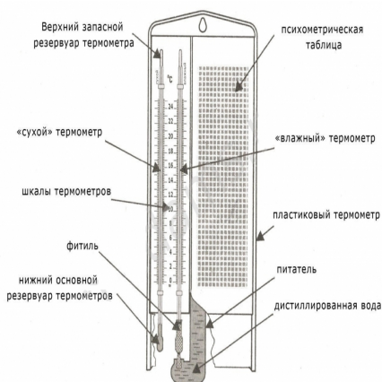
Рис. 37. Психрометр Августа
