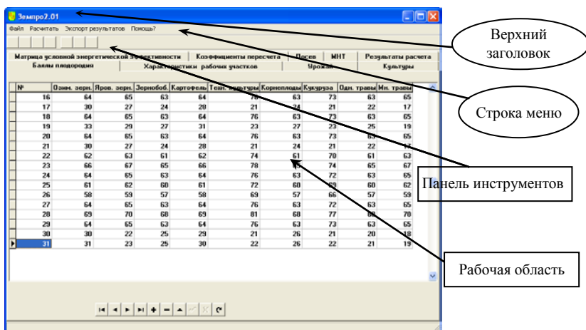
Рис. 3.1. Интерфейс программы Zepro
