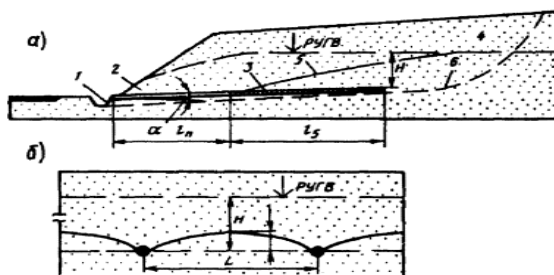
Рисунок 2. – Схема бестраншейного горизонтального дренажа:
