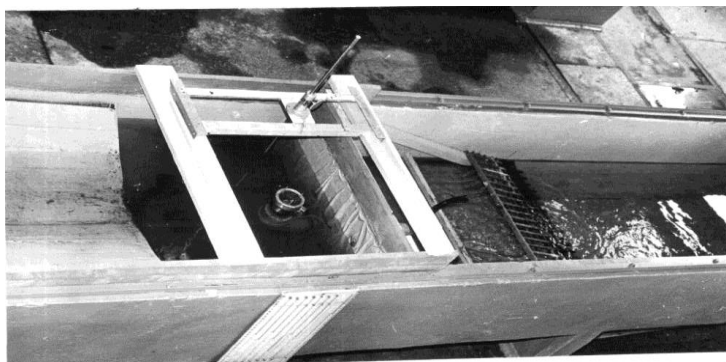
Рисунок 1. – Модель экспериментальной установки
