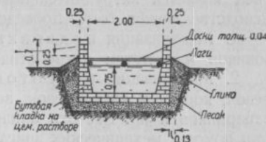
Рис. 120. Поперечный разрез купальни.
