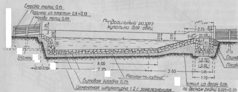
Рис. 119. Продольный разрез купальни.
