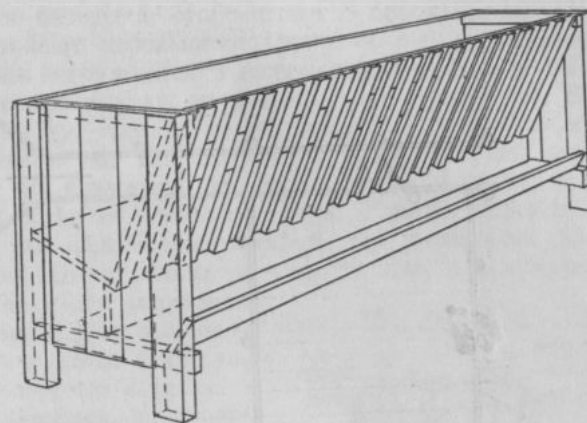
Рис. 116. Стенные ясли для сена и зерна.
