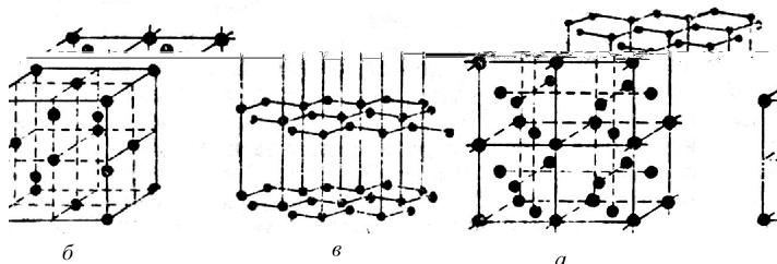
Рис. 1.1. Кристаллические решетки некоторых минералов: a – медь – спайность отсутствует; б – алмаз – спайность, совершенная в четырех направлениях; в – графит – спайность весьма совершенная
