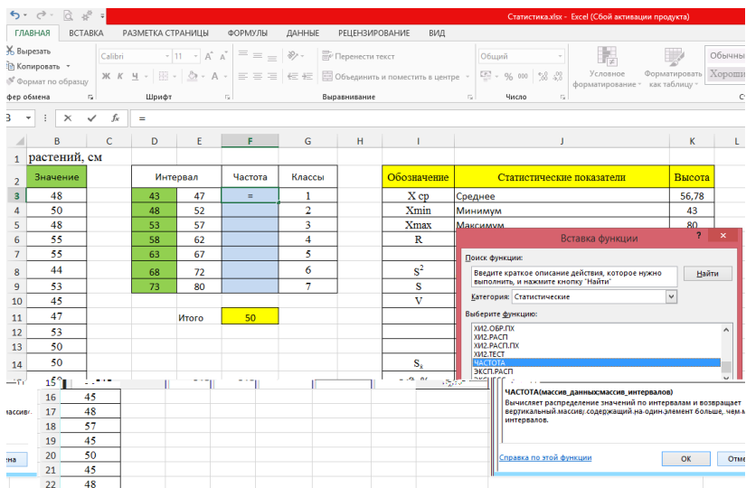
Рис. 2. Пример распределения частот
