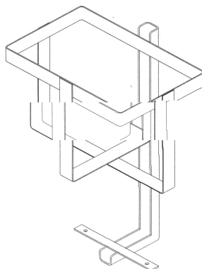
Рис. 20. Кассета
