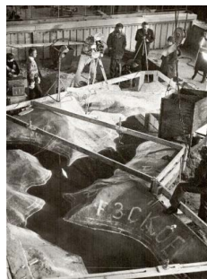
Рис. 3. Модельные исследования волновых режимов в Сарезском озере вследствие обвалов и оползней
