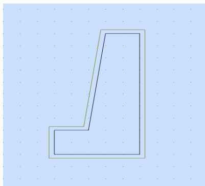
Рис. 2. Контур профиля подпорной стенки
