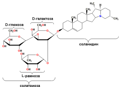
Рис. 1. Строение соланидина
