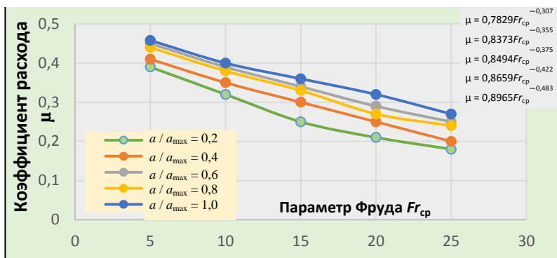
Рис. 3. Зависимости коэффициентов расхода от параметра Фруда: а – ВДКБТ-АР; б – ВДКБТ-АП
