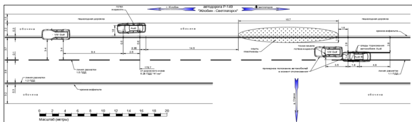
Рис. 4. Реальные конечные положения автомобилей после совершения дорожно-транспортного происшествия
