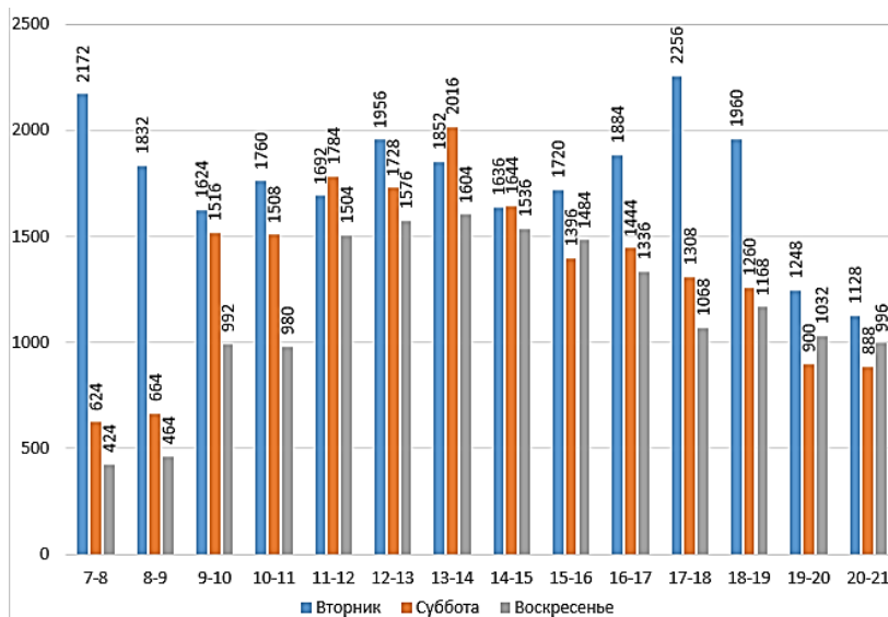
Рис. 2. Диаграмма распределения транспортных потоков по дням недели и часам суток
