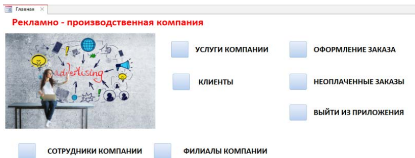
Рис. 2. Главная форма
