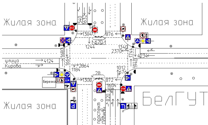
Рис. 1. Цифрограмма интенсивностей движения во вторник с 7:00 до 20:00 суммарно (авт/14 час, пеш/14 час)
