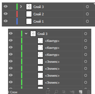
Рис. 1. Слой
