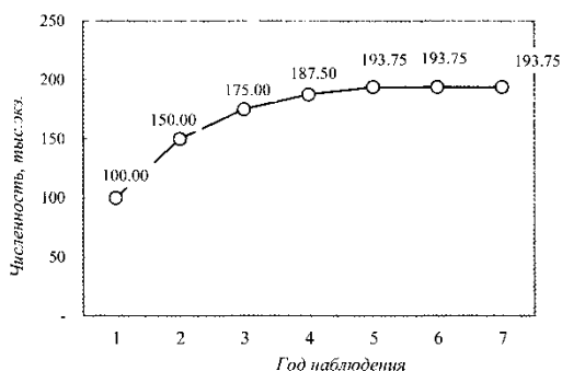
Рис. 4. Схема формирования общей численности популяции
