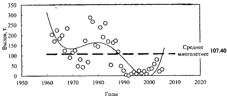
Рис. 19. Регрессионный прогноз вылова
