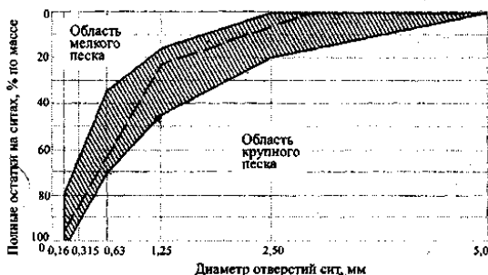
Рис. 6.1. График зернового состава песка
