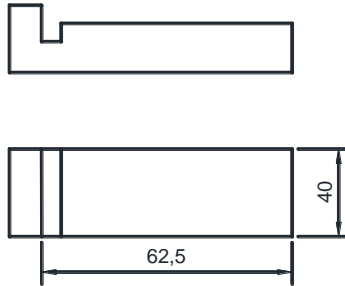
Рис. 4.17. Стальные пластинки для испытания на сжатие половинок балочек
