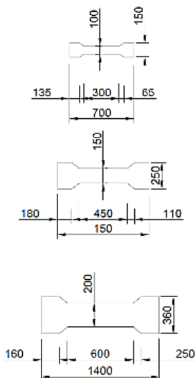
Рис. 7.3. Образцы-восьмерки
