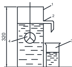
Рис. 1.3. Объемомер: 1 – металлический цилиндр; 2 – латунная трубка; 3 – стакан; 4 – испытуемый образец
