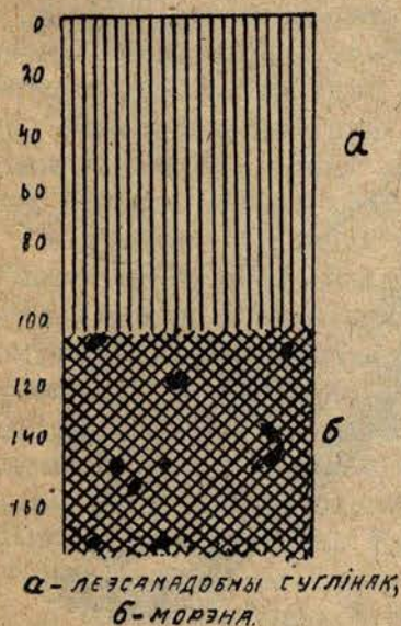
Мал. 6.—Моцна падзолавая глеба на лёсападобным суглінку
