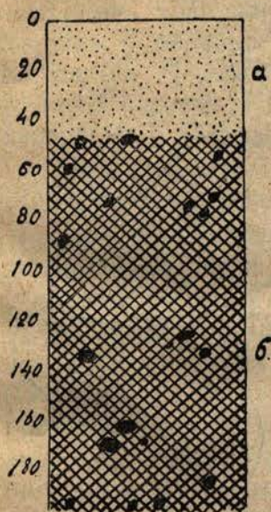
а - пухкі пясок б - марэна
