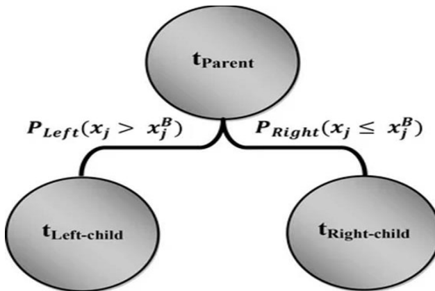
Рис. 6.1. Дерево решений по алгоритму CART
