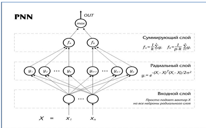
Рис. 5.6. Нейронная сеть PNN
