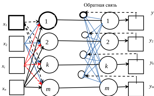
Рис. 5.5. Нейронная сеть Хэмминга
