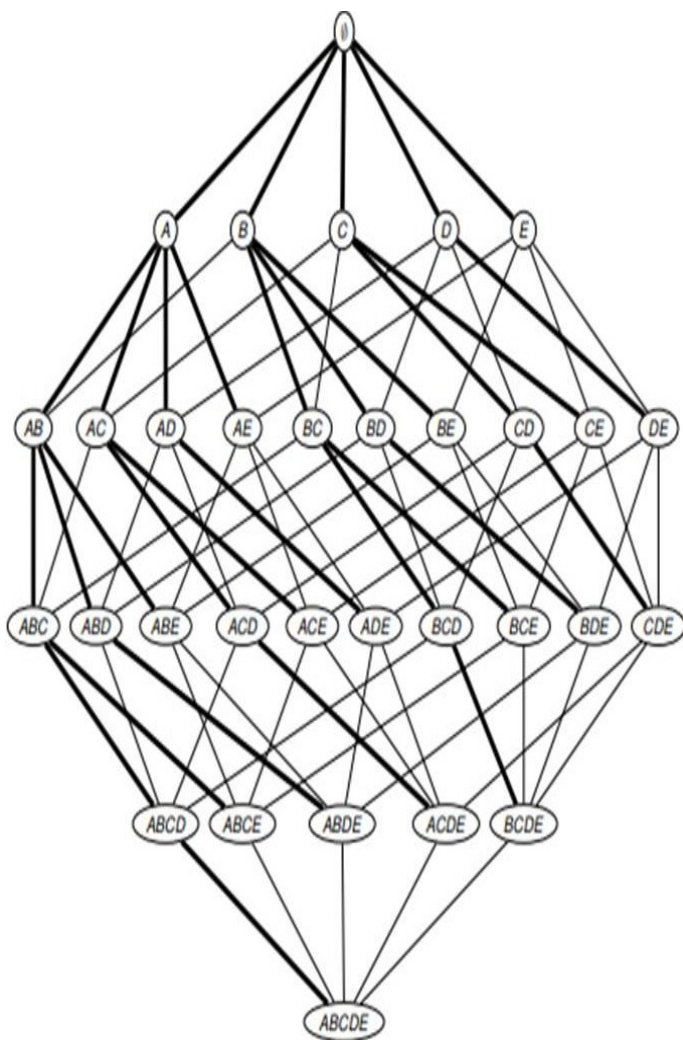
Рис. 8.1. Алгоритм Apriori
