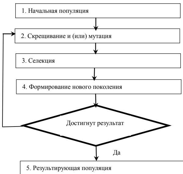
Рис. 14.3. Алгоритм эволюции
