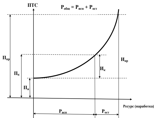
Рис. 6.1. Схема определения остаточного моторесурса машин и оборудования: R_{исп} – использованный ресурс к моменту контроля; I_k – изменение значения параметра к моменту контроля (диагностирования); I_{пр} – предельное изменение значения параметра; R_{ост} – остаточный ресурс
