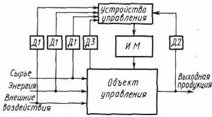
Рис. 1.6. Упрощенная схема управления технологическим процессом
