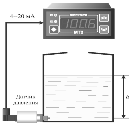
Рис. 3.3. Гидростатический уровнемер
