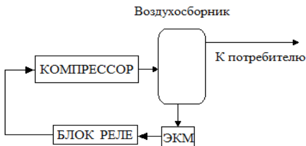
Рис. 10.4. Структурная схема автоматизации компрессора
