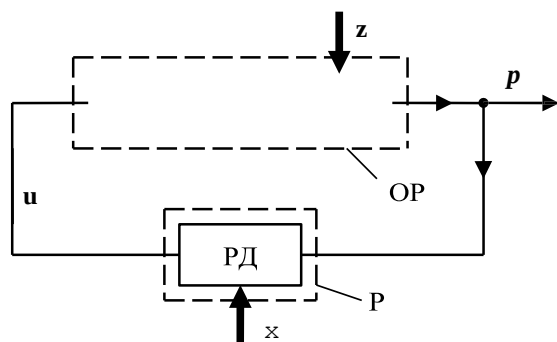
Рис. 9.1. Функциональная схема САР с регулированием по давлению
