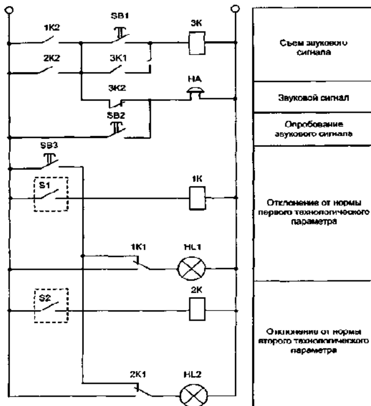
Рис. 1.2. Схема сигнализации
