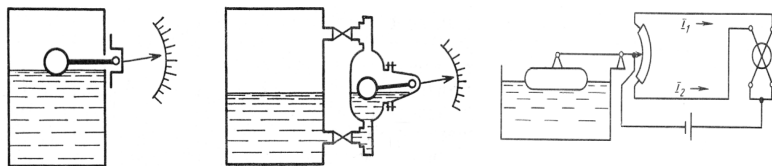
Рис. 3.6. Примеры поплавковых уровнемеров
