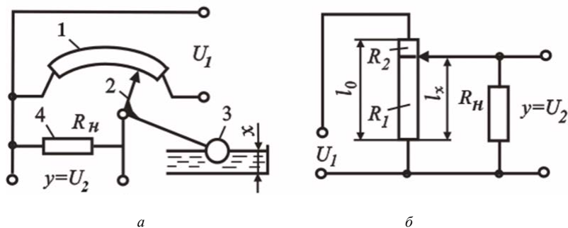
Рис. 2.1. Схемы потенциометрического датчика:
