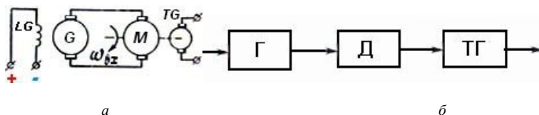
Рис. 1.7. Схема электропривода: а – принципиальная; б – структурная
