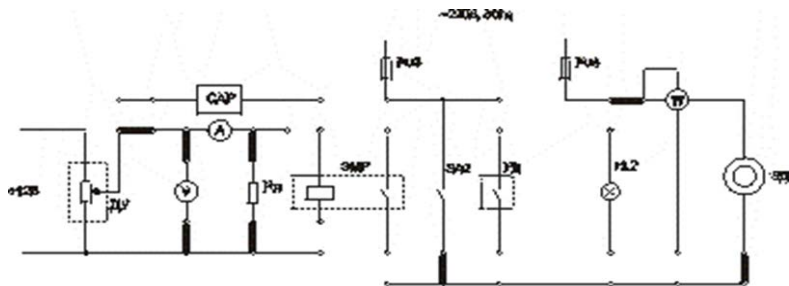
Рис. 2.5. Схема электрических соединений
