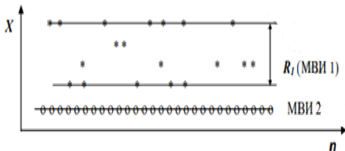
Рис. 5.2. Точечные диаграммы двух серий многократных измерений
