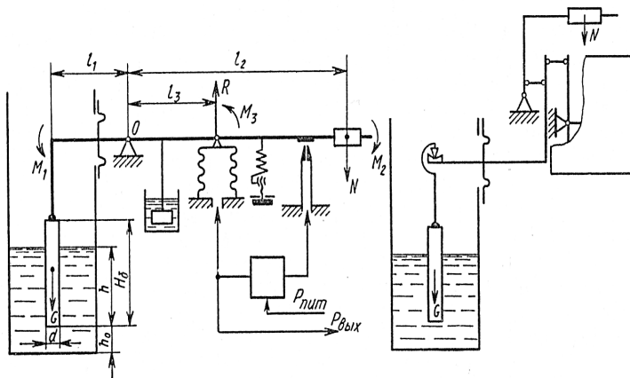
Рис. 3.4. Буйковые уровнемеры
