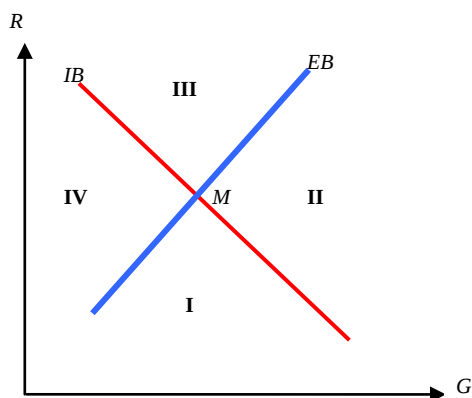
Рис. 9.3. Диаграмма Свона
