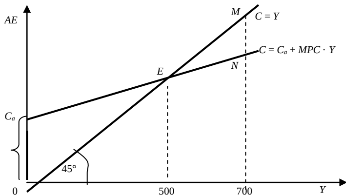
Рис. 3.2. Функция потребления
