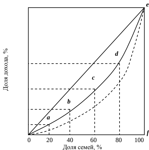
Рис. 11.1. Кривая Лоренца
