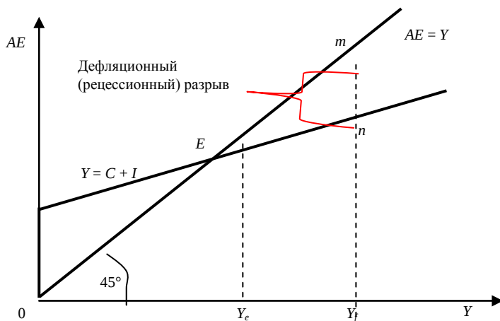
Рис. 3.11. Дефляционный разрыв
