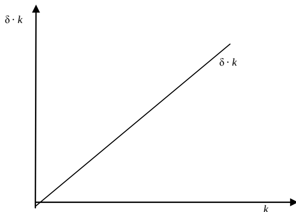
Рис. 10.4. Выбытие капитала
