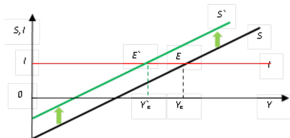
Рис. 3.10. Парадокс бережливости
