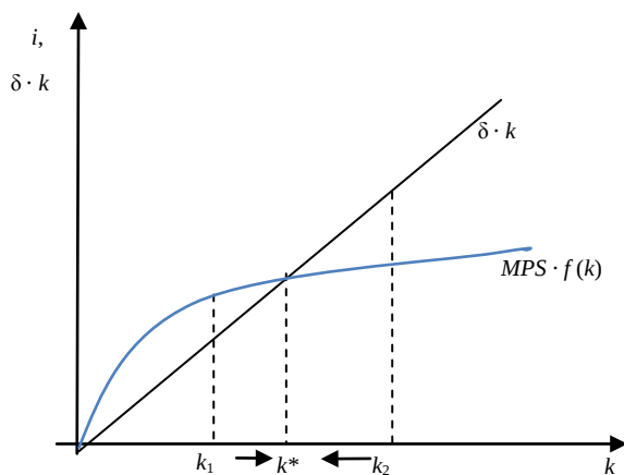
Рис. 10.5. Капиталовооружённость
