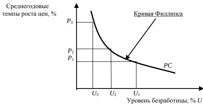
Рис. 7.3. Кривая Филлипса
