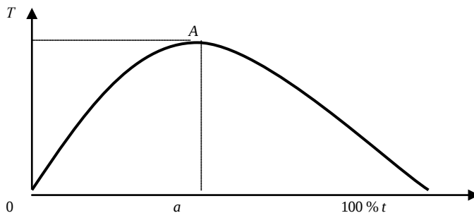
Рис. 7.7. Кривая Лаффера
