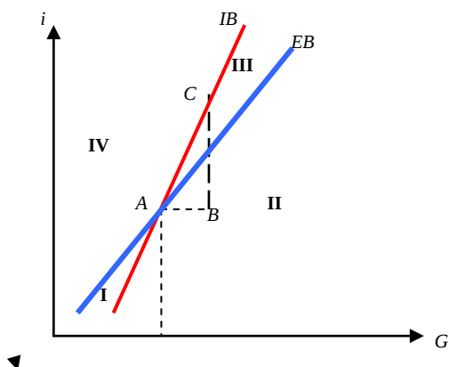
Рис. 9.4. Модель Манделла
