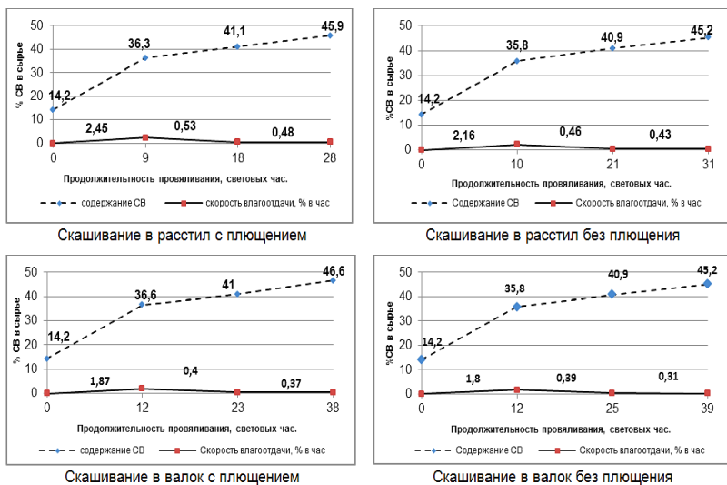
Рис. 5. Продолжительность и скорость проявляния галеги восточной в фазу стеблевания при разных технологических приемах
