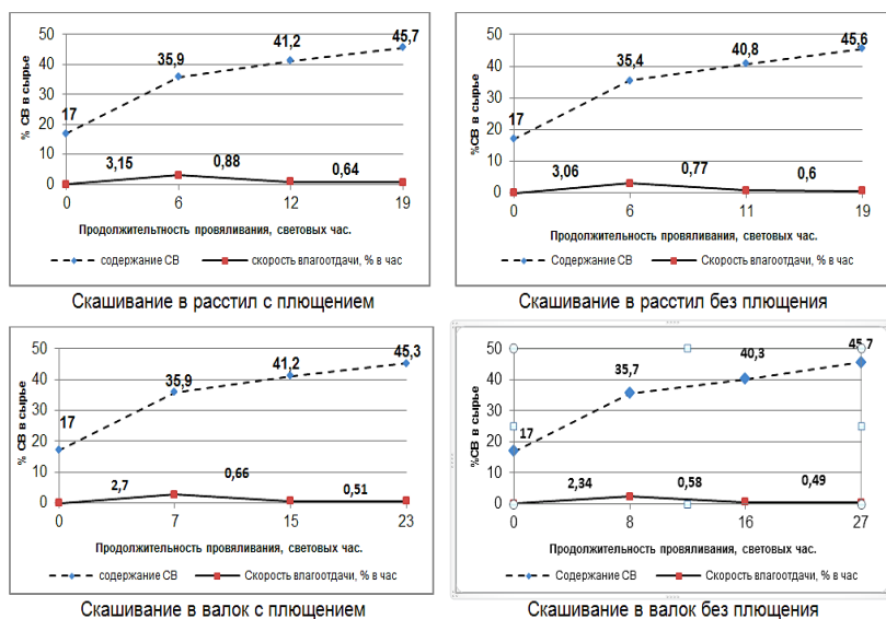
Рис. 2. Продолжительность и скорость проявлявания клевера лугового в фазу бутонизации при разных технологиях
