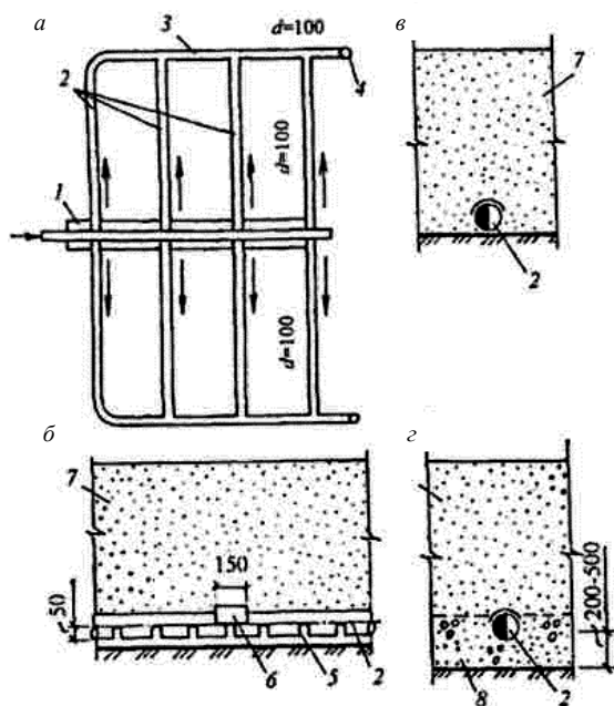
Рис. 6.16. Поля подземной фильтрации: а – план; б – продольный разрез; в – поперечный разрез; г – то же, при укладке на слой щебня шлака или крупного песка; 1 – распределительный лоток оросительной трубы; 2 – оросительные трубы; 3 – вентиляционный коллектор; 4 – вентиляционный стояк; 5 – пропилы; 6 – рубероид толь, промасленная бумага и т. п.; 7 – засыпка из местного грунта; 8 – засыпка щебнем, шлаком или крупным песком
