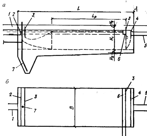
Рис. 6.8. Горизонтальный отстойник: а – разрез; б – план; 1 – подводящий лоток; 2 – распределительный лоток; 3 – полупогружные доски; 4 – сборный лоток; 5 – отводной лоток; 6 – лоток для сбора и удаления плавающих веществ; 7 – трубопровод для удаления осадка
