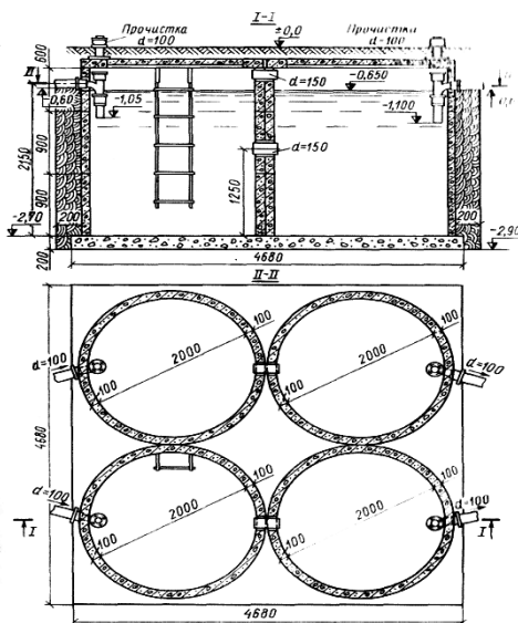
Рис. 6.10. Многокамерный септик из железобетонных колец
