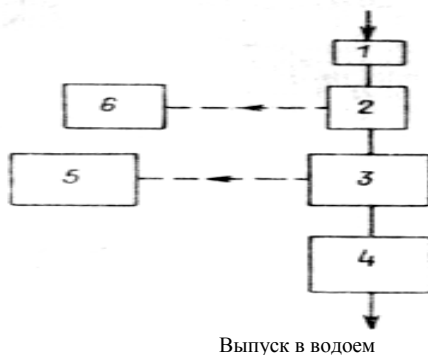
Рис. 6.2. Схема станции с биологической очисткой сточных вод:
