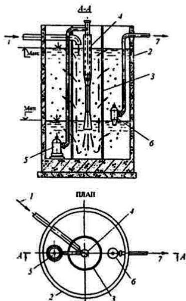
Рис. 6.20. Установка «Контакт»: 1 – подача сточной жидкости; 2 – емкость азротенка; 3 – центральная цилиндрическая сетка; 4 – эжекторный азратор; 5 – циркулярный насос; 6 – насос для откачки очищенных сточных вод; 7 – выпуск очищенной воды
