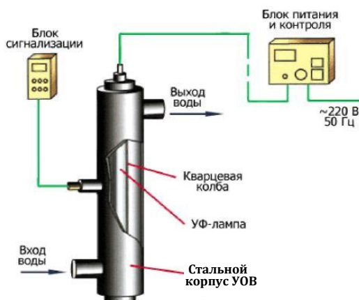
Рис. 6.24. Принципиальная схема ультрафиолетовой установки для обеззараживания воды
