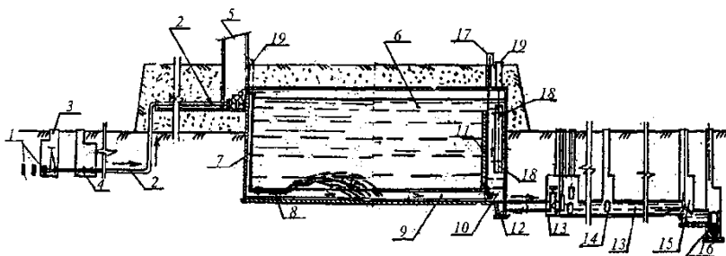
Рис. 5.7. Принципиальная высотная схема расположения АРР по отношению к подводящему каналу НС: 1 – напорные водоводы от НС; 2 – трубопровод, подающий воду в галерею задвижек; 3 – колодец с задвижками; 4 – колодец с расходомером; 5 – галерея задвижек с регулирующими устройствами; 6 – аварийно-регулирующий резервуар; 7 – подающая в АРР труба; 8 – эжектор с коническим насадком на подводящей к АРР трубе; 9 – лотковая часть днища АРР; 10 – водосборный канал; 11 – поперечная перегородка с водопропускным проемом; 12 – приямок опорожнения АРР; 13 – труба опорожнения АРР с запорно-регулирующими устройствами; 14 – канал опорожнения АРР с колодцами на присоединении от смежных секций АРР; 15 – водоизмерительный пост на канале опорожнения АРР; 16 – колодец; 17 – фильтр-поглотитель; 18 – переливная труба АРР; 19 – лазы в АРР
