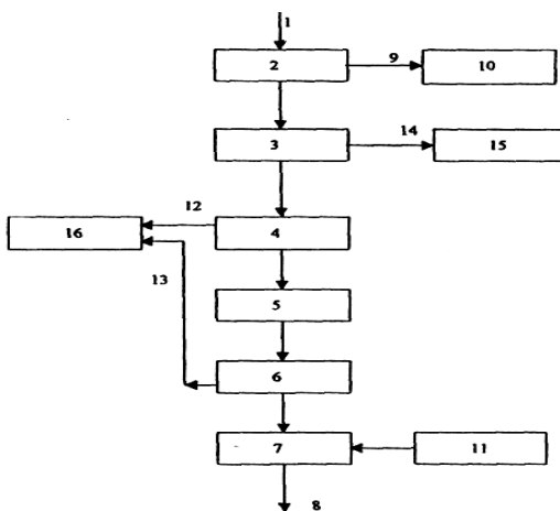
Рис. 6.3. Технологическая схема очистной станции с биологической очисткой сточных вод на биофильтрах:
