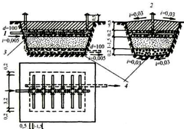
Рис. 6.18. Песчано-гравийный фильтр: 1 – подача осветленной сточной жидкости; 2 – вентиляционная труба; 3 – оросительная сеть; 4 – дренажная сеть
