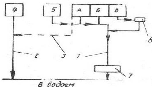
Рис. 4.19. Схема раздельной системы водоотведения с местными очистными установками: A, B, B – цехи (производственные воды); 1 – сеть бытовых и загрязненных производственных сточных вод; 2 – сеть дождевых вод; 3 – выпуск условно чистых производственных вод; 4 – дождевые воды; 5 – бытовые воды; 6 – местные очистные установки; 7 – очистная станция
