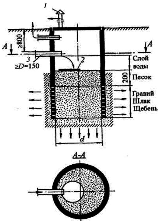
Рис. 6.15. Фильтрующий колодец: 1 – вентиляционная труба; 2 – отражающая плита; 3 – подача осветленной сточной жидкости
