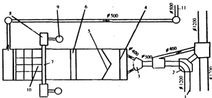
Рис. 4.27. Очистные сооружения камерного типа: 1 — подводный коллектор; 2 — разделительная камера; 3 — вход осветляемой воды; 4 — переливная стенка; 5 — решетка; 6 — плавучий понтон; 7 — сборник нефтепродуктов; 8 — нефтесепараторная камера; 9 — слив воды; 10 — фильтры доочистки; 11 — отвод очищенной воды
