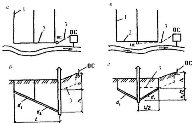
Рис. 5.2. Схемы водоотведения города с одной насосной станцией (а, в) и продольные профили главных коллекторов (б, г): 1 – коллекторы; 2 – главные коллекторы; 3 – напорные трубопроводы
