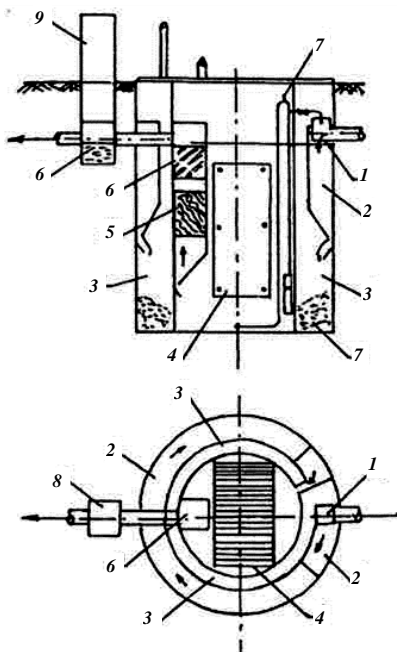
Рис. 6.19. Компактный блок очистных сооружений (КБС): 1 – решетка; 2 – остойный желоб; 3 – сбраживатель; 4 – азротенк с плоскостным инертным наполнителем; 5 – осветлитель с тонкослойным отстаиванием; 6 – высокопористый фильтр; 7 – погружной насос с эжектором; 8 – контактный резервуар; 9 – шкаф системы КИПиА и обеззараживания
