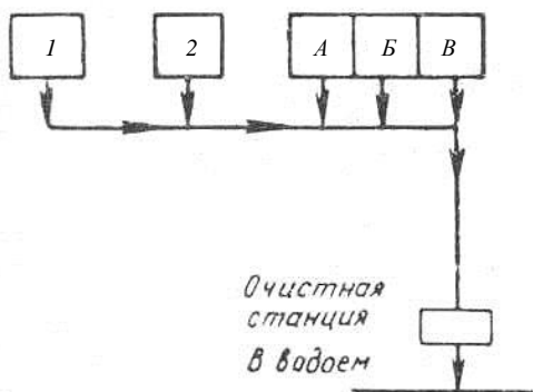
Рис. 4.18. Схема общесплавной системы водоотведения: A, B, B – цехи (производственные воды); 1 – дождевые воды; 2 – бытовые воды
