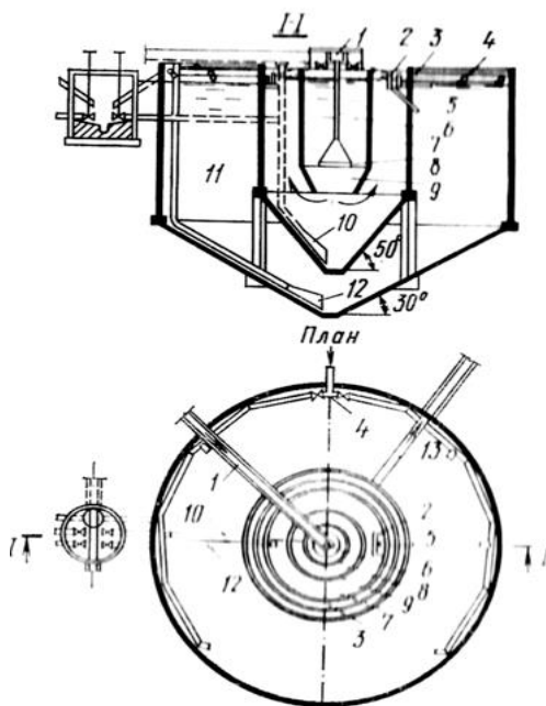
Рис. 6.11. Осветлитель-перегиватель:
