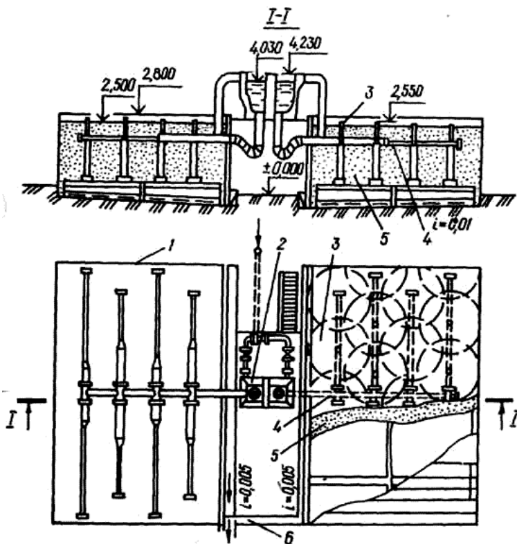
Рис. 6.9. Биофильтр:
