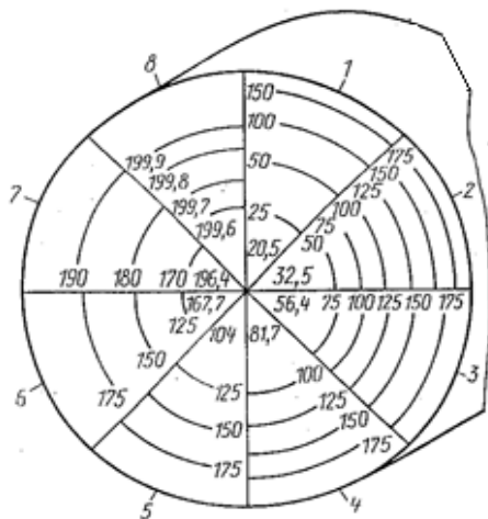
Рис. 2. Распределение температурных полей по толщине наплавляемого слоя при нанесении износостойких покрытий ЭМН для сплошных круглых сечений
