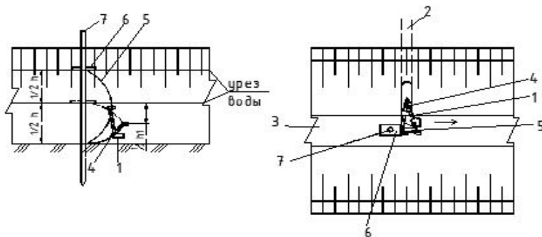
Рис. 2. Устье коллектора с поплавковой г-образной насадкой: 1 – устье; 2 – дренажный коллектор; 3 – канал; 4 – гибкий патрубок; 5 – эластичная диафрагма; 6 – поплавок; 7 – направляющая штанга
