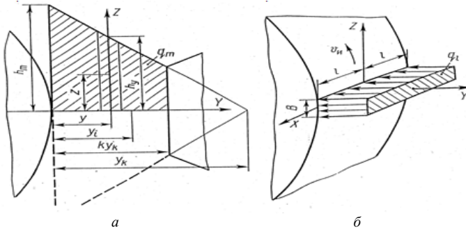
Рис. 1. Расчетная схема для определения температурных полей в рабочей зоне линейного теплоисточника при нанесении покрытий электромагнитной наплавкой
