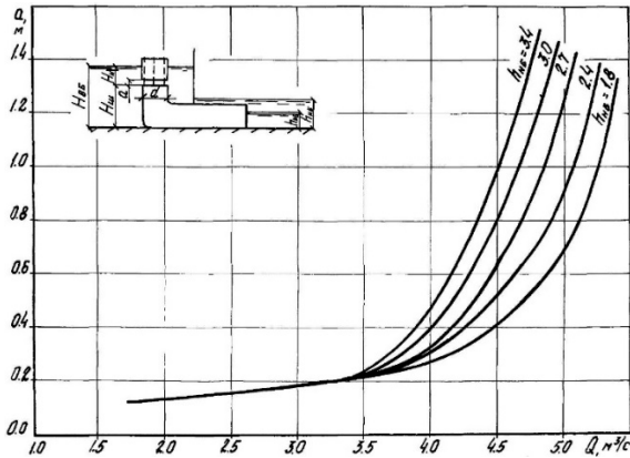
Рис. 3. Графики пропускной способности Q = f(a; h_{нб}) для d = 1,2 м H_{вб} = H_1 = 6,0 м и высоты шахты H_{ш} = 4,5 м
