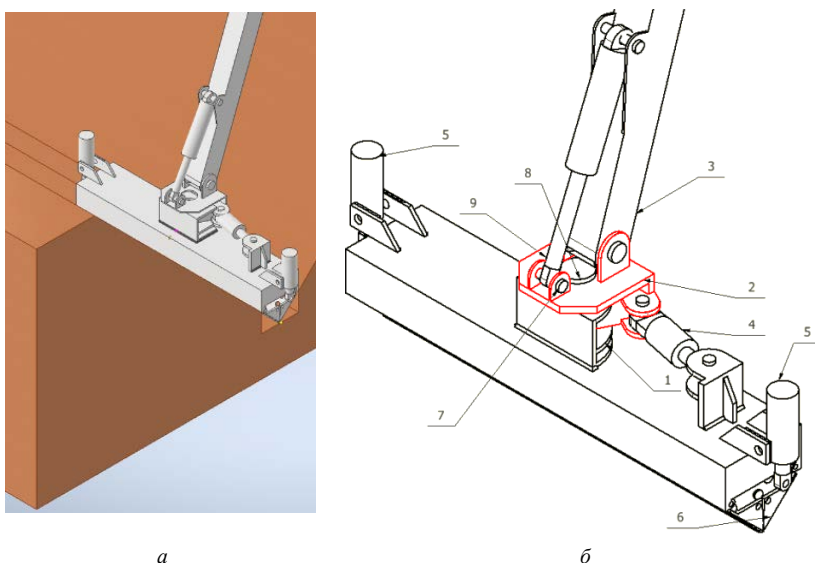
Рис. 2. Предлагаемый уширенный ковш к каналоочистителю ОКН-0,5: а – в работе; б – конструктивные элементы ковша
