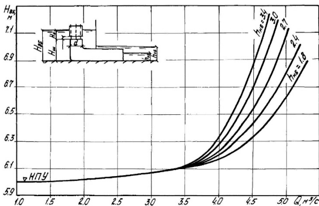
Рис. 2. Графики пропускной способности Q = f(H_{\text{ВБ}}; h_{\text{нб}}) для d = 1,2 м, H_{\text{ВБ}} = H_1 = 6,0 м и высоты шахты H_{\text{ш}} = 4,5 м
