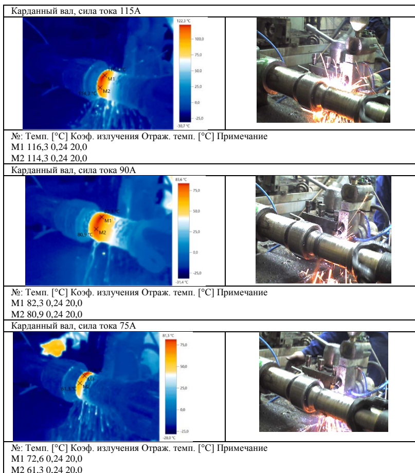
Рис. 3. Термограммы ЭМН карданного вала трубчатого сечения
