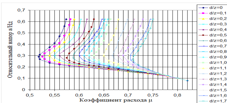
Рис. 2. Коэффициенты расхода водосброса \mu_{\text{н}} = f(a / H_{\text{д}})
