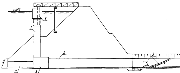
Рис. 1. Башенный водосброс с поплавковым затвором
