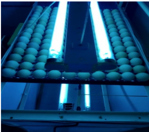
Рис. 1. Обработка инкубационных яиц ультрафиолетовым излучением С-спектра на экспериментальной установке
