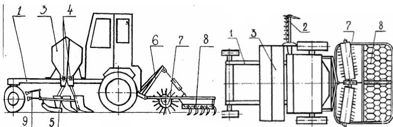
Рис. 2. Схема комбинированного агрегата для ухода за пастбищами: 1 – самоходное шасси; 2 – косилка; 3 – сеялка; 4 – высевающие аппараты; 5 – сошники; 6 – задняя навеска; 7 – игольчатая борона; 8 – пастбищная борона
