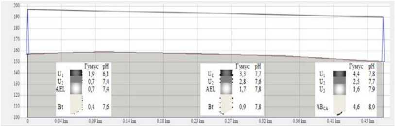
Рис. 1. Содержание гумуса и pH почвенного раствора в профилях катены арматурный завод – пойма р. Бык
