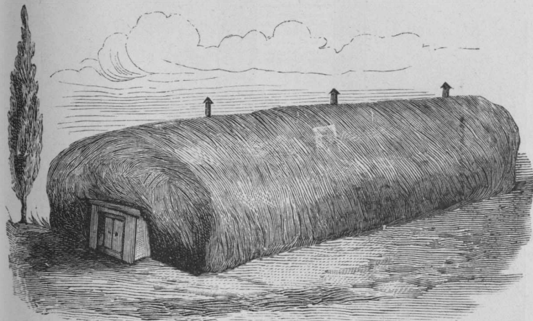
Рис. 22. Наружный видъ плодохранилища В. Таурскаго.
