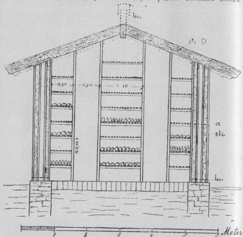
Рис. 38. Поперечный разрѣзъ Гейзенгеймскаго плодохранилища.
