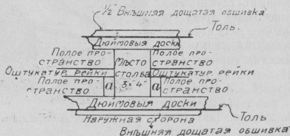
Рис. 29. Устройство стѣны въ плодохранилищѣ Кинней.
