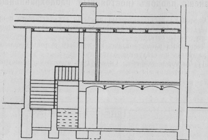
Рис. 13. Разрѣзъ плодового погреба Штольце по линіи а В (рис. 12).
