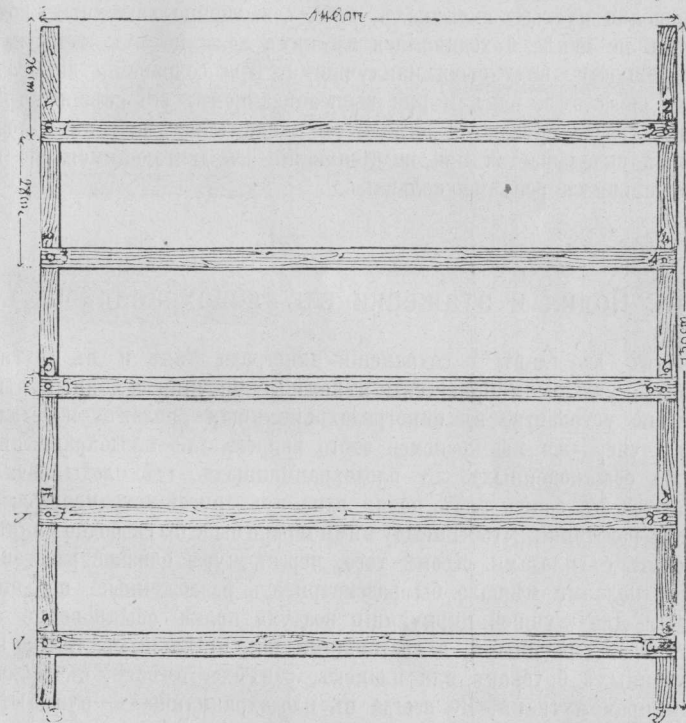
Рис. 70. Видъ спереди стѣнки плодовой шкафной этажерки Гегелювена.
