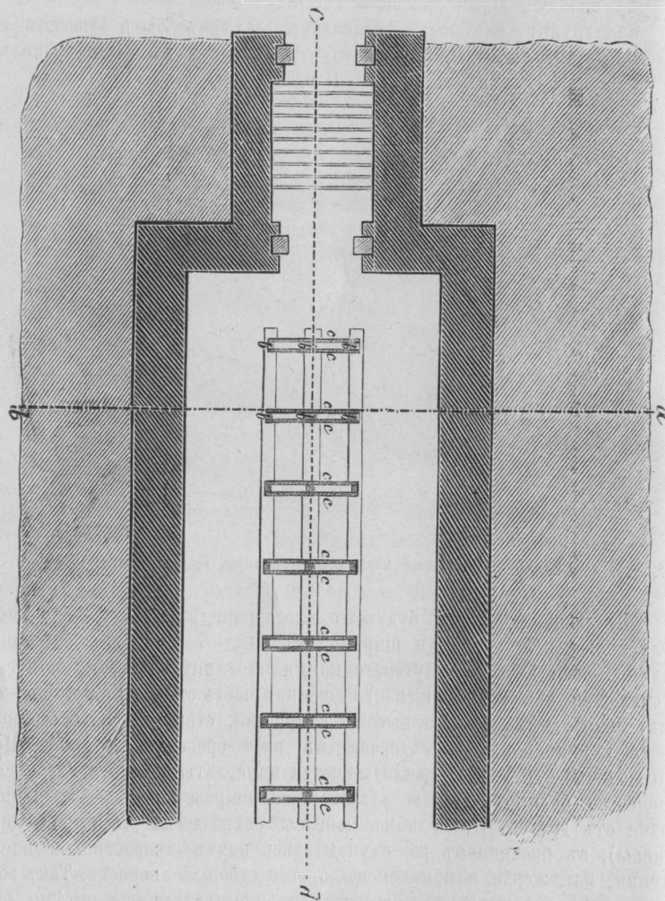
Рис. 23. Планъ плодохранилища В. Таюрскаго.
