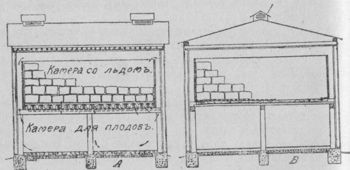
Рис. 45. Продольный и поперечный разрѣзы постройки для храненія льда въ верхнемъ этажѣ и плодовъ въ нижнемъ.
