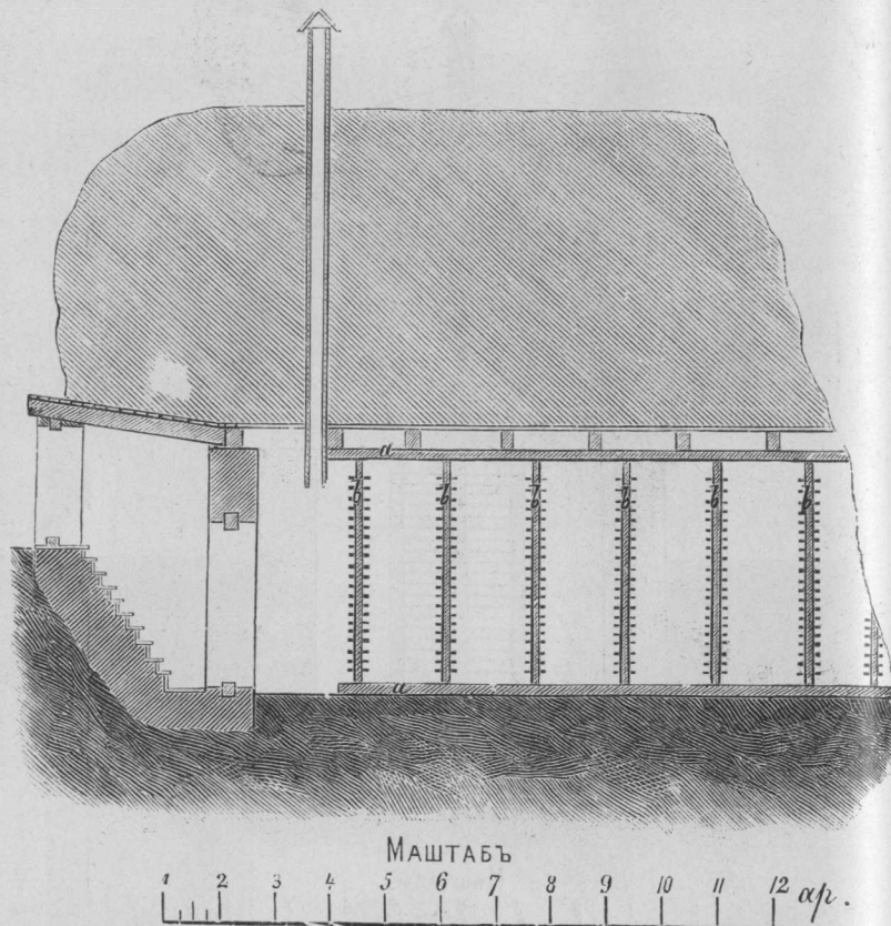
Рис. 25. Прочный разрезъ плодохранилища В. Таюрскаго.
