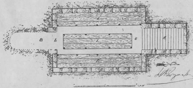
Рис. 87. Планъ овощнаго лабаза въ с. Бѣляевкѣ подъ Одессой.
