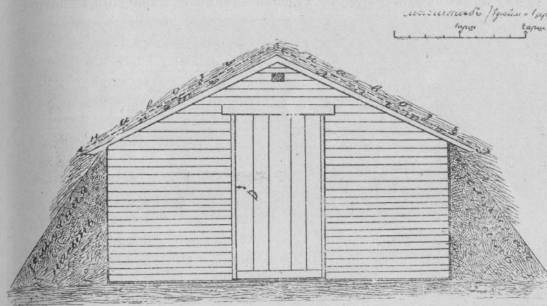
Рис. 26. Фасадъ надземнаго плодохранилища г. Трусова.
