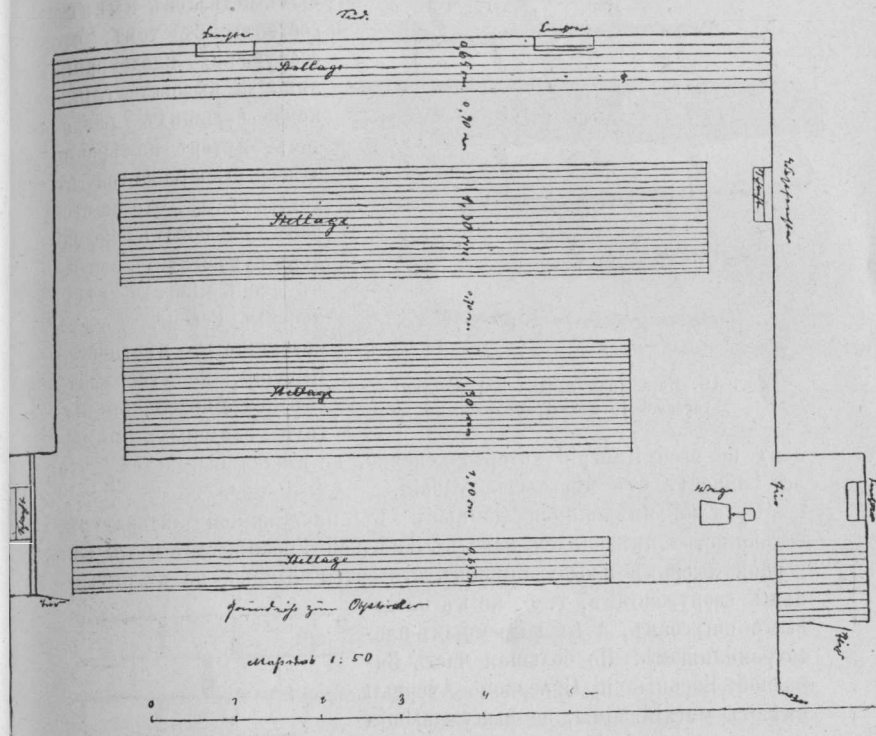
Рис. 15. Планъ Саксентаузенскаго плодохранилища.
