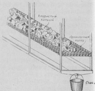
Рис. 7. Способъ устройства полокъ для кальція.
