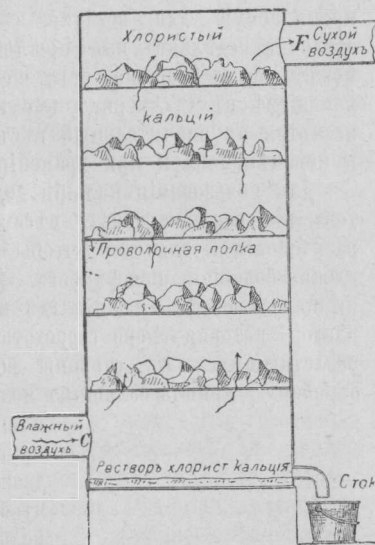
Рис. 8. Приспособленіе для осушенія воздуха въ плодохранилищахъ.
