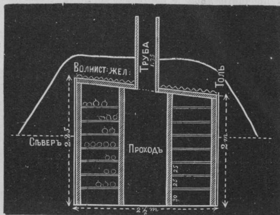
Рис. 20. Поперечный разрыв землянки Вебера.
