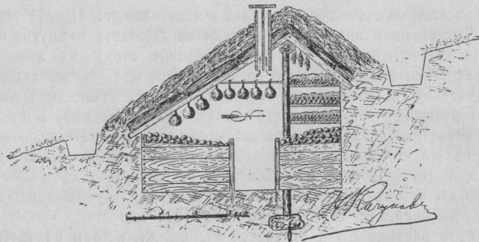
Рис. 86. Разрѣзъ овощнаго лабаза подъ Одессой съ деревяннымъ потолкомъ.
