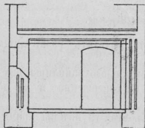
Рис. 14. Поперечный разрѣзъ плодохранилища Штольце.
