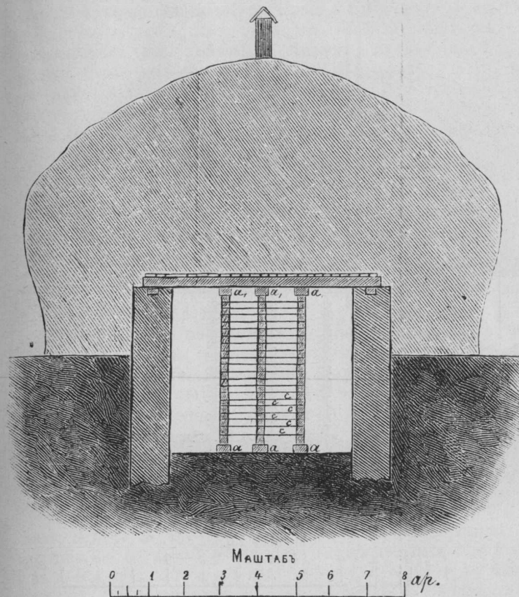
Рис. 24. Поперечный разрѣзъ плодохранилища В. Таюрскаго.
