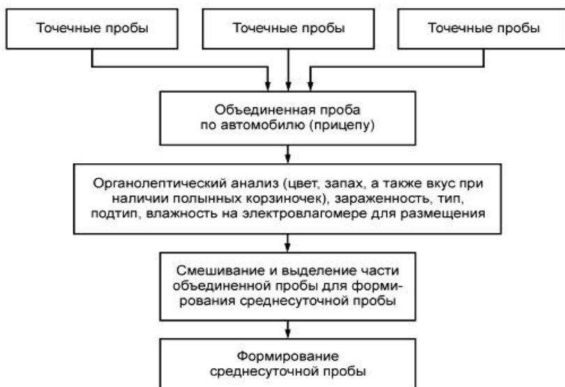
Рис. 2. Схема формирования среднесуточной пробы
